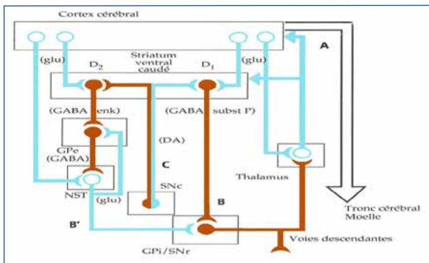
Figure 2 - Circuiterie fonctionnelle du système des ganglions de la base. Influences excitatrices (noir), influences inhibitrices (gris). Neurotransmetteurs : glu (glutamate), DA (dopamine), enk (enképhaline). D1 et D2 désignent les deux types de récepteurs à la dopamine. GPe (Globus Pallidus externe), GPi (Globus Pallidus interne), SNc (Substance Noire pars compacta), SNr (Substance Noire pars reticulata), NST (noyau subthalamique). Boucle cortico-thalamo-corticale (A), boucles directe et indirecte (B et B'), boucle nigro-striée (C).
