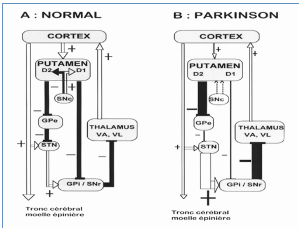
Figure 3 - Situation normale et pathologique dans la maladie de Parkinson. Influences excitatrices (noir), influences inhibitrices (gris). Globus pallidus externe (GPe), globus pallidus interne (GPi), noyau subthalamique (STN), substance noire pars reticulata (SNr), substantia nigra pars compacta (SNc), thalamus ventrolatéral (VL). D1 et D2 désignent les deux types de récepteurs à la dopamine.
