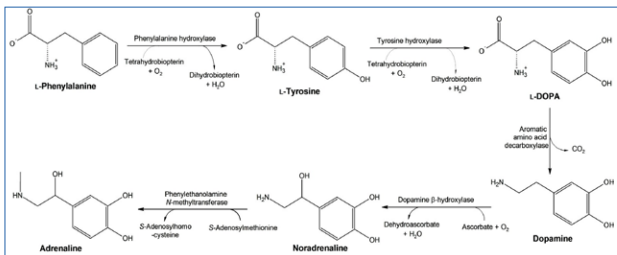
Figure 1 - Métabolisme des catécholamines. Les voies métaboliques de synthèse des catécholamines partent de deux acides aminés essentiels la Phénylalanine et la Tyrosine, la tyrosine étant le produit de la phénylalanine hydroxylase. Une tyrosine hydroxylase oxyde à nouveau le cycle aromatique pour produire la dihydroxyphénylalanine (DOPA). Une DOPA décarboxylase produit la dopamine, qui est ensuite oxydée en noradrénaline, puis méthylée en adrénaline.
