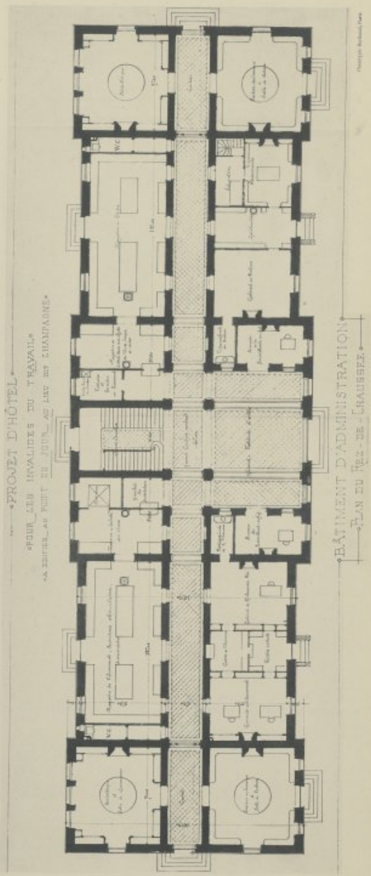
HÔTEL DES INVALIDES DU TRAVAIL, A LYON. - 1. Vue du bâtiment d'administration. - 2. Plan du Bas-de-Chaussée (Bâtiment d'administration). M. Henri MONODOR, Architecte à Lyon.
