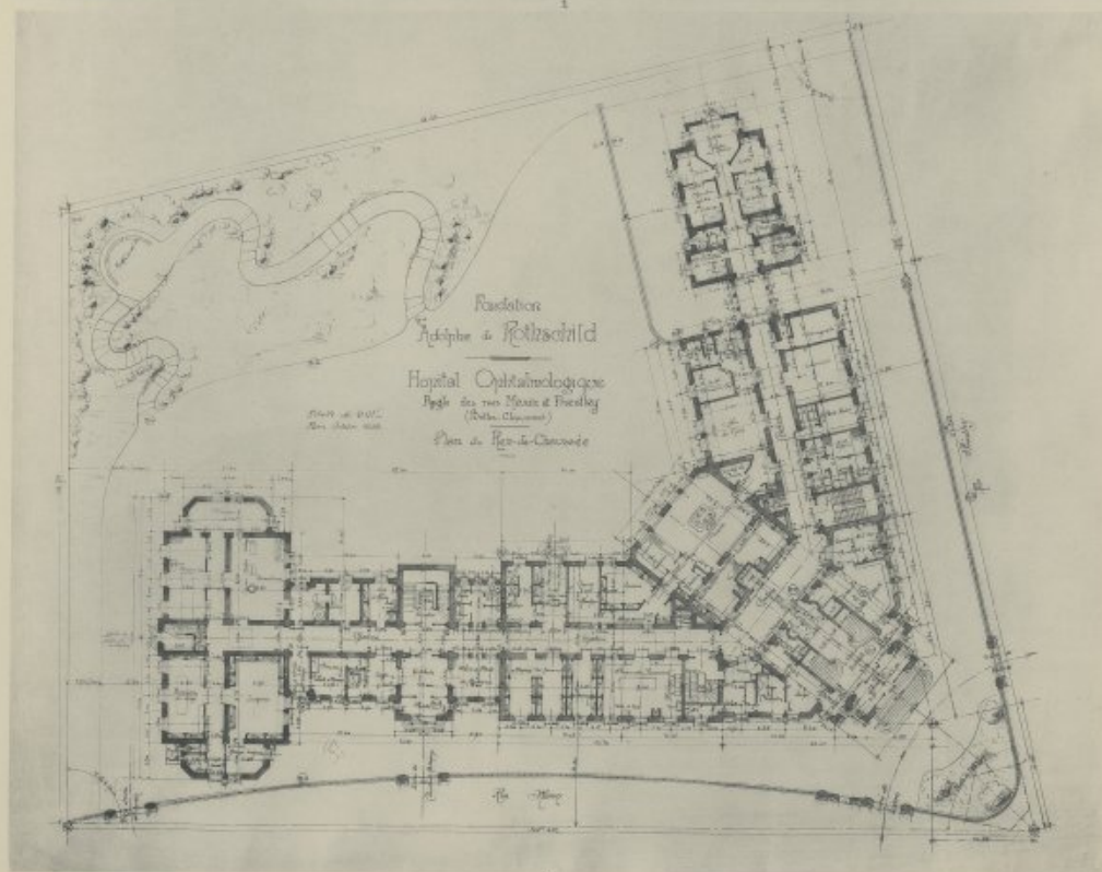
HOPITAL OPHTALMOLOGIQUE A. DE ROTHSCHILD, A PARIS. - 1. Plan du 1 er Etage. - 2. Plan du Rez-de-Chaussée. MM. CHATENAY et ROUTRE, Architectes à Paris.
