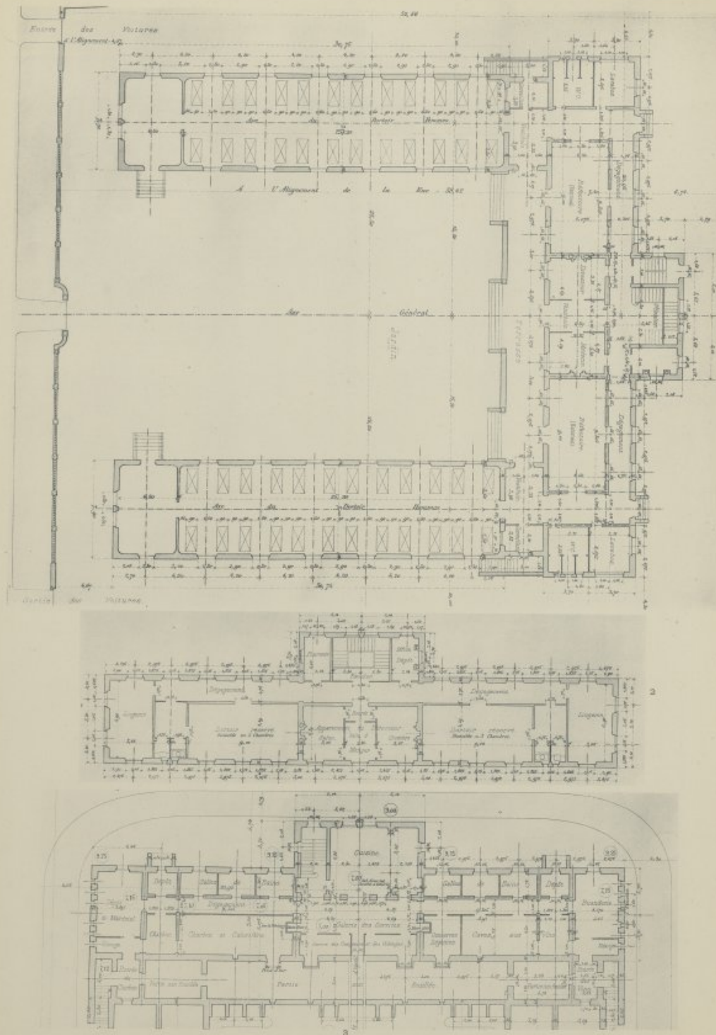
MAISON MUNICIPALE DE VIEILLARDS (FONDATION VALENTIN) A LEVALLOIS-PERRET. 1. Plan du Rez-de-Chaussée - 2. Plan du 1 er Étage - 3. Plan du Sous-Sol. MM. KUPFER ET LEPEIGNEUX, Architectes à Paris.
