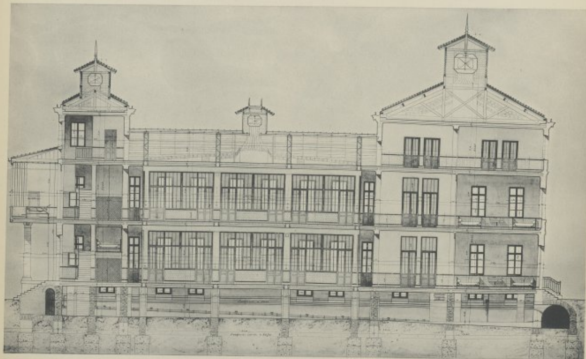
HOPITAL DE L'INSTITUT PASTEUR, A PARIS. - 1. Coupes transversales - 2. Coupe longitudinale. M. FLORENTIN-MARTIN, Architecte à Paris.
