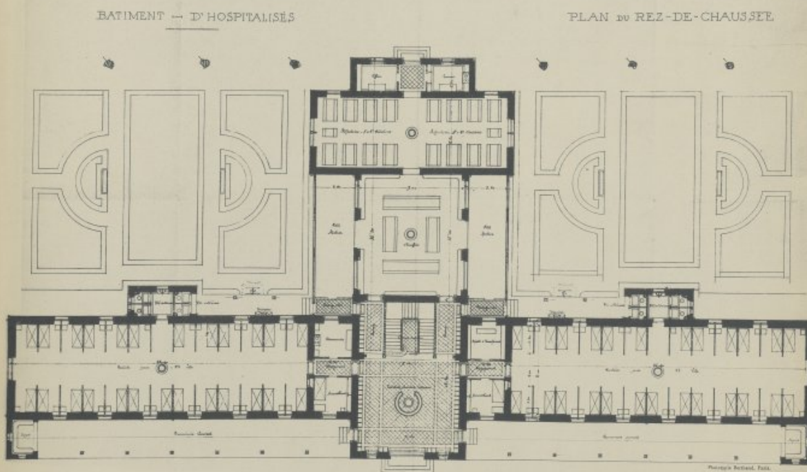
HOTEL DES INVALIDES DU TRAVAIL, A LYON. — 1. Vue d'un bâtiment d'hospitalisés. — 2. Plan du Rez-de-Chaussée (Bâtiment d'hospitalisés). M. Henri MONCORGÉ, Architecte à Lyon.
