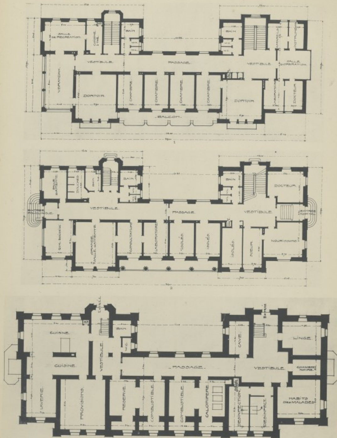
HOPITAL D'ENFANTS ET DISPENSAIRE DE GUENWILLER (Alsace). — 1. Plan du 1 er Etage — 2. Plan du Rez-de-Chaussée. 3. Plan du Sous-Sol. M. C. SCHULE, Architecte (MM. Seltzer et Schule), à Mulhouse.
