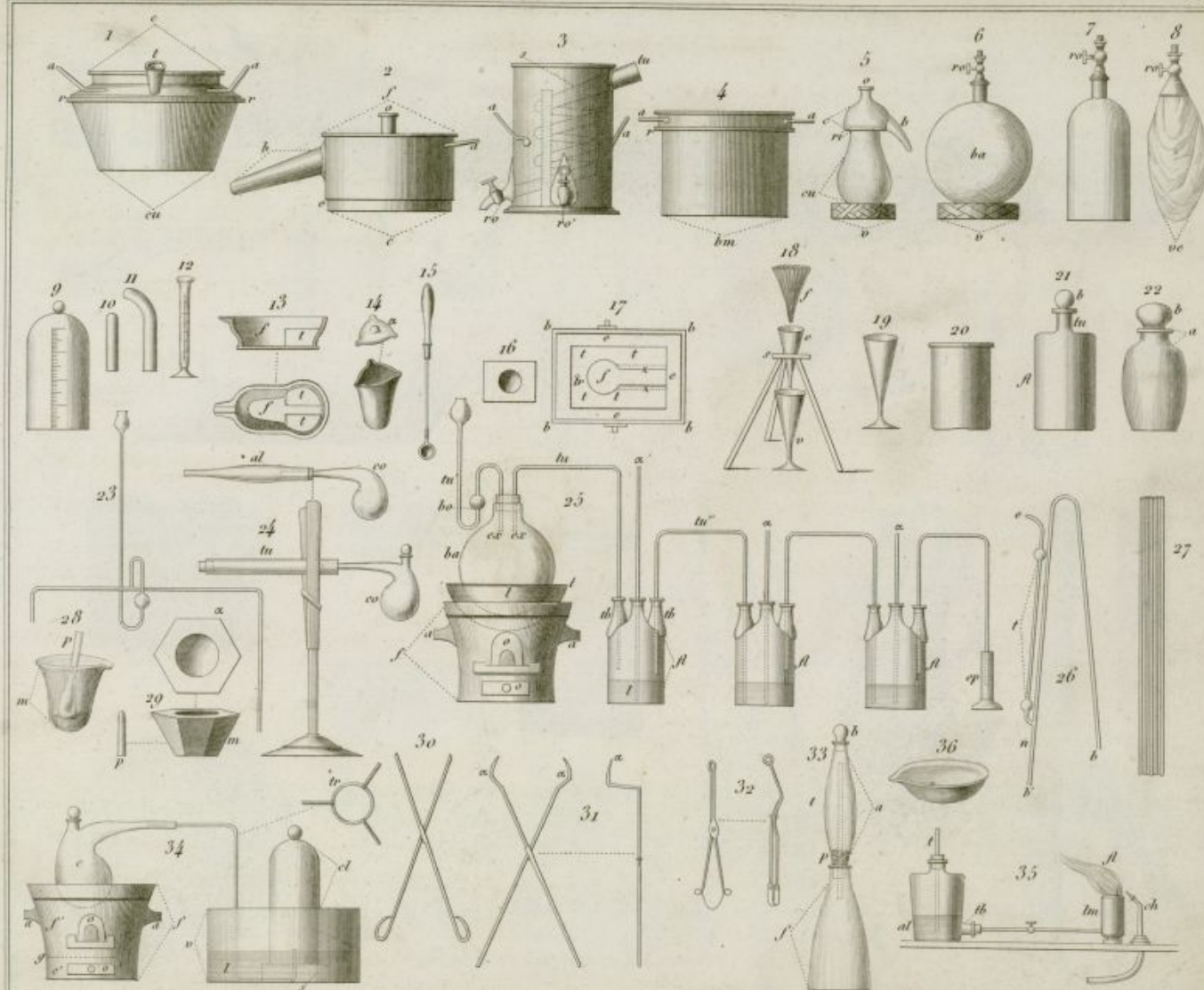
Appareils des manipulations en grand.
