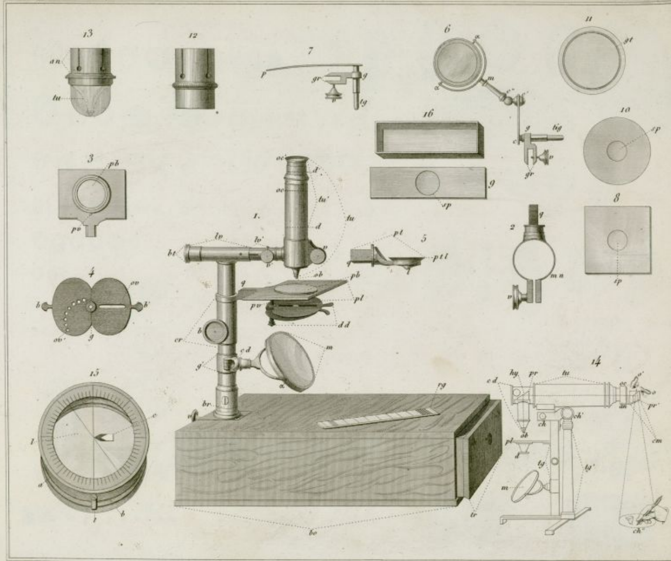
1 a 13 Microscope double. — 14 Microscope horizontal. 15 Goniomètre microscopique.
