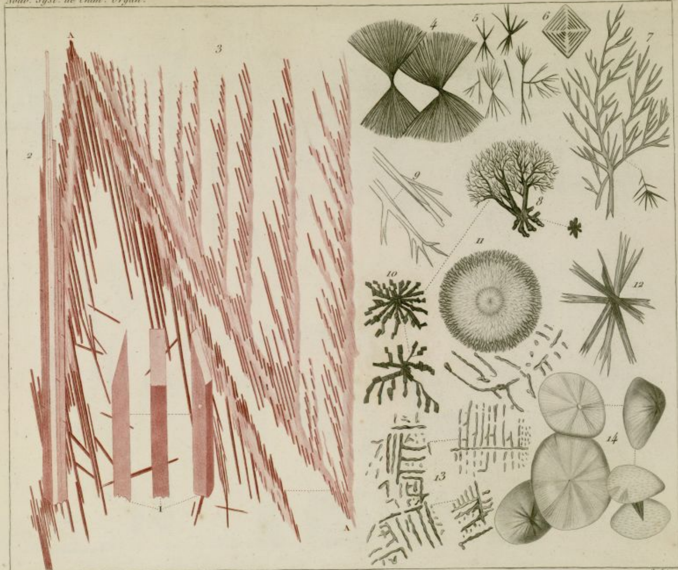
1, 2, 3 matière colorante de la garance — 4, 5, 7 quinine — 6 chlorate de potasse — 9, 11, 12, narcotine. — 8, 10 carbonate de soude. — acétate d'ammoniaque. — acétate et sous acétate de plomb.
