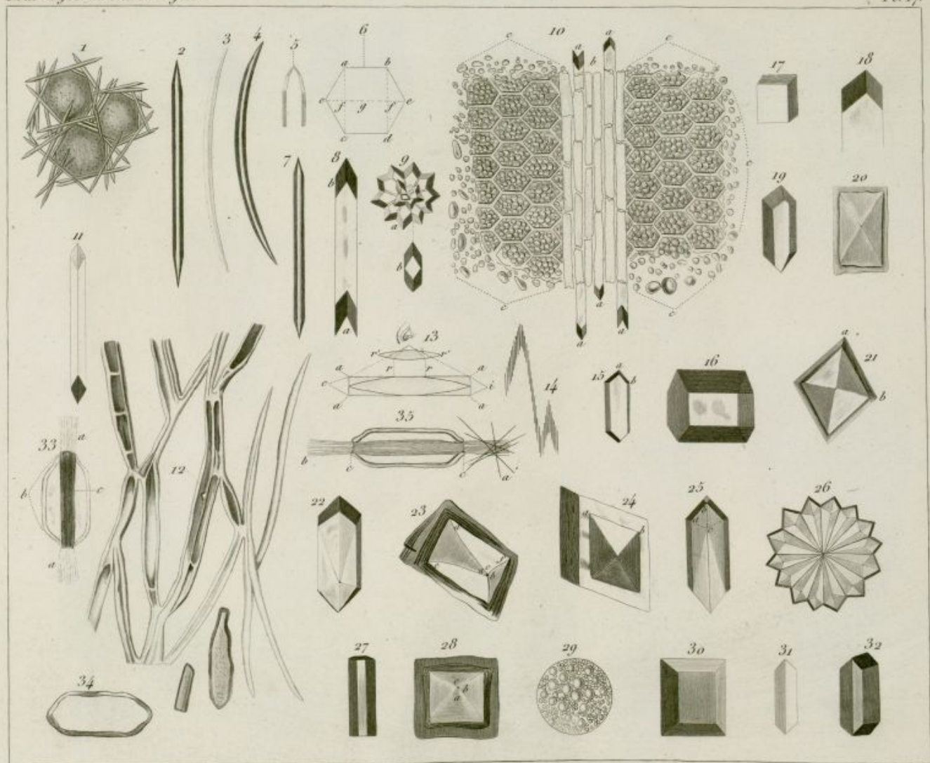
Études microscopiques de la Cristallisation.
