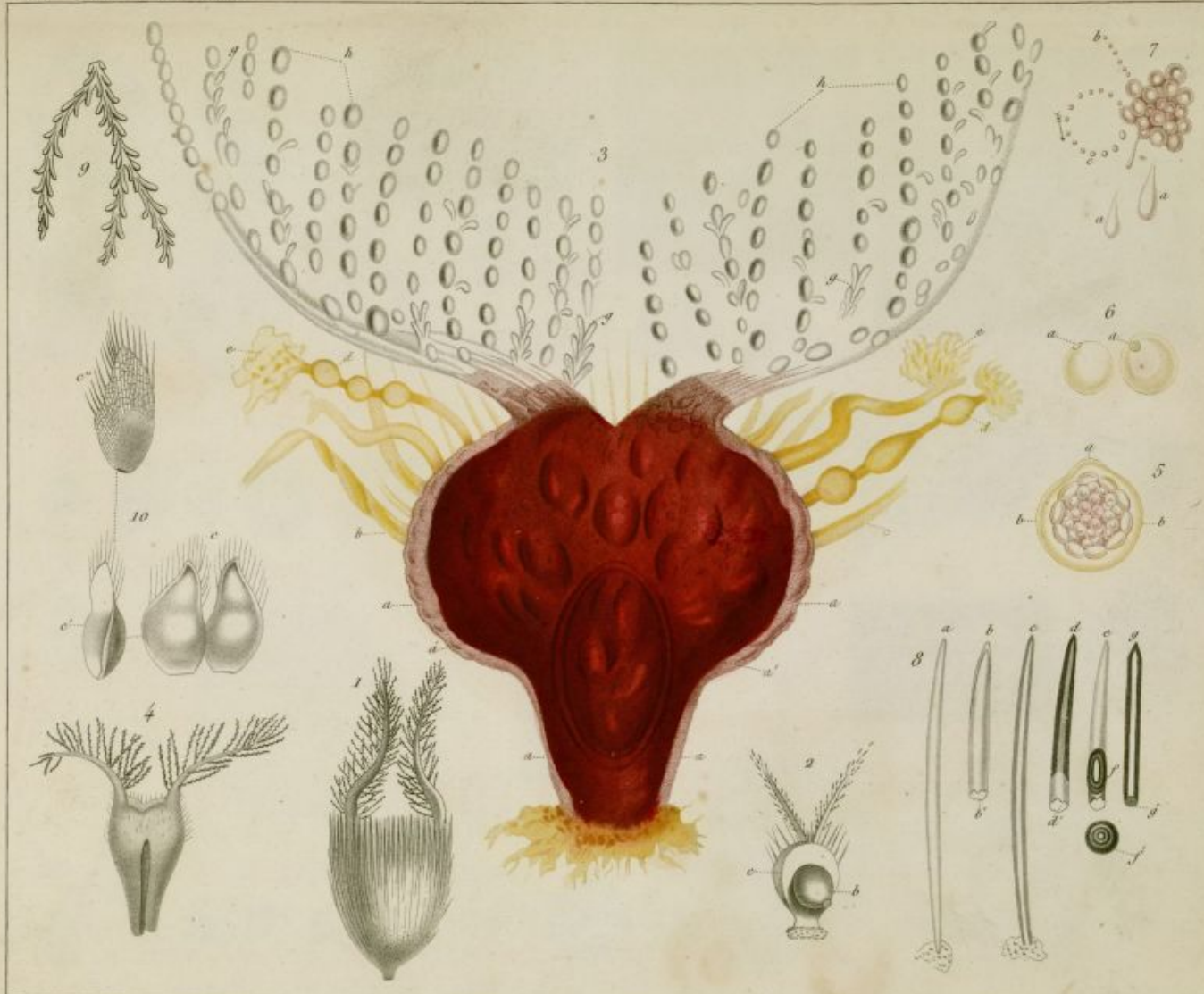
Réactif du Sucre de l'Albumine et de l'Huile.
