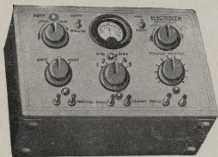
Appareil "Electrocecm" indispensable en Médecine générale
