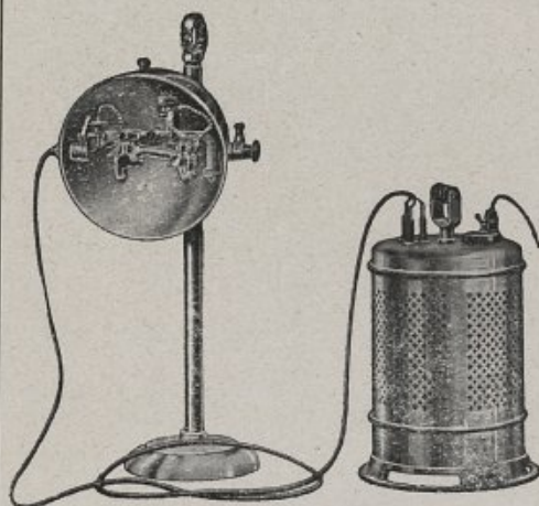
M. 600 Lampe U.-V. portable
