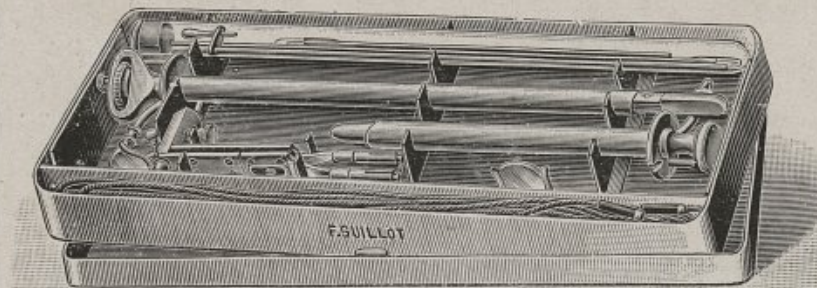
F. 435 CYSTOSCOPE de Luys, à vision directe, complet en boîte métal avec 2 tubes, pour urètre masculin et féminin, cordons, lampe, etc. 3500. »
