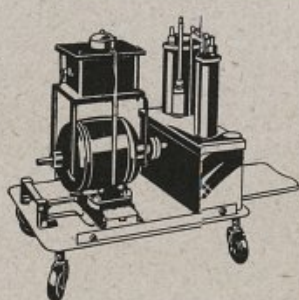
M. 110 Aspirateur chirurgical (voir ci-dessus) Sans son capot
