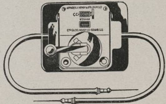
B. 413 Appareil de Jouvet.
