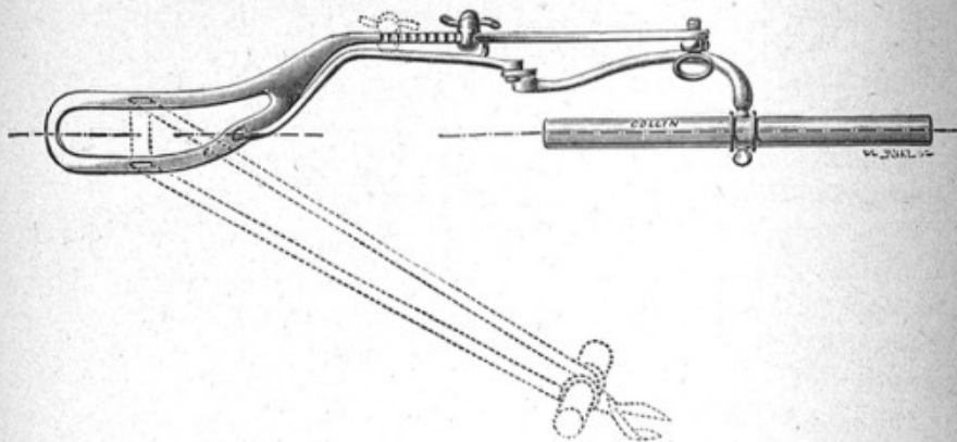
Fig. 3. — Forceps-levier construit de manière à comparer les tractions au centre de figure et celles qu'effectue le système de Tarnier-modifié. (Les lacs, dessinés en pointillé, sont volontairement écartés de l'axe de traction, pour plus de clarté.)
