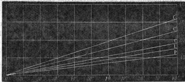
Fig. 26. — Les temps sont comptés sur l'axe des abscisses, à raison de 6 centimètres à l'heure; chaque expérience a duré 1 h. 40 minutes. Les calories se comptent sur l'axe des ordonnées, à raison de 1 millimètre par calorie. — P, courbe calorigraphique de la poule; L, du lapin; C, du chat; C', du chien; C'', des Cobayes.
