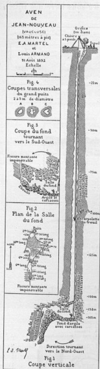
FIG. 10. — Abîme à désobstruer (pour accéder aux réservoirs de Vaucluse).
