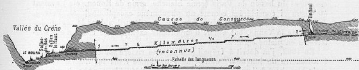
Fig. 29. — Origine des cascades de tufs de Salles-la-Source (Aveyron). Mise en liberté, à l'air libre, du carbonate de chaux sursaturant une rivière souterraine d'un plateau calcaire.
