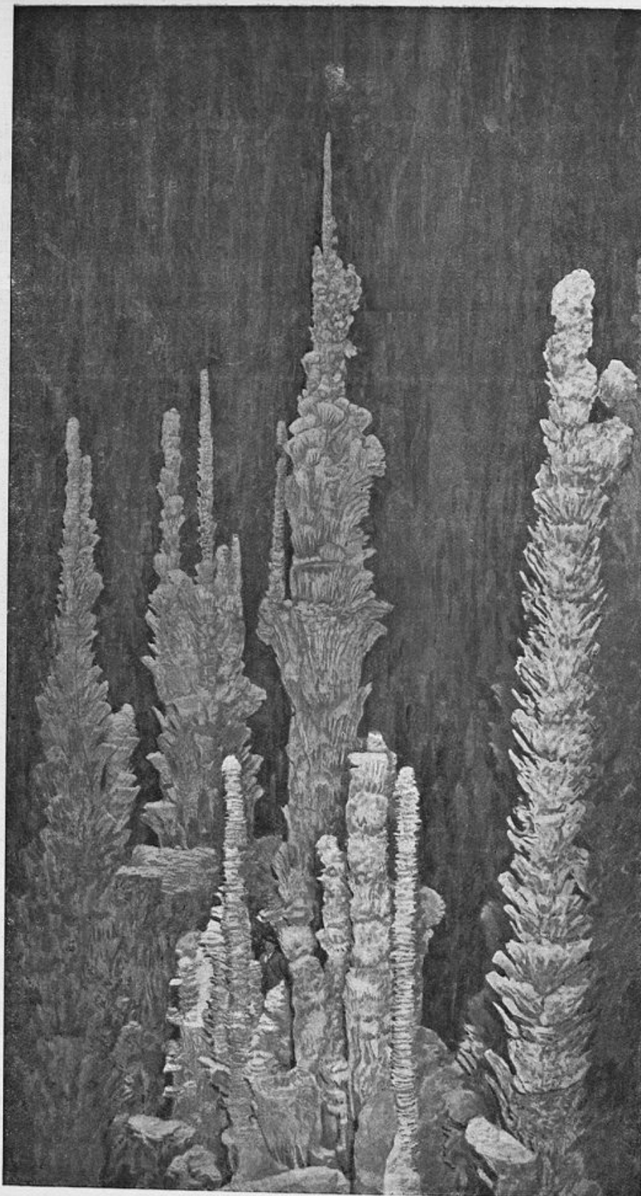
FIG. 46. — Spécimen de photographie au magnésium (grandissement de 2 clichés 8×9 raccordés). La grande stalagmite (hauteur 30 mèt.) de l'Aven-Armand (Lozère).
