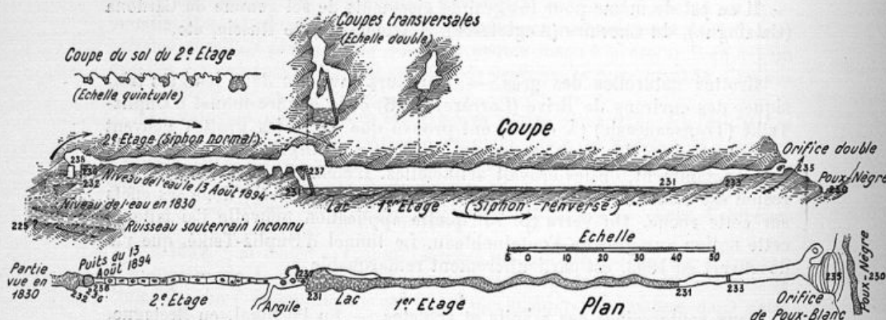
FIG. 30. — Coupe et plan expliquant le mécanisme du trop plein rémittent d'une émergence calcaire (Poux-Blanc, Tarn-et-Garonne). (P. 63.)
