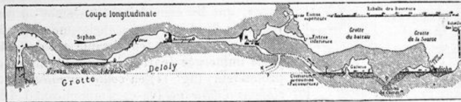
FIG. 11. — Exemple de siphons désamorçés en temps de sécheresse (sources de l'Écluse, Ardèche, 1892).
