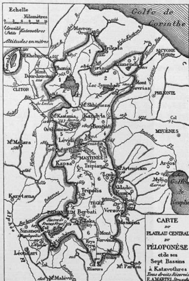
FIG. 43. — Katavothres du Péloponèse (V. p. 95).
