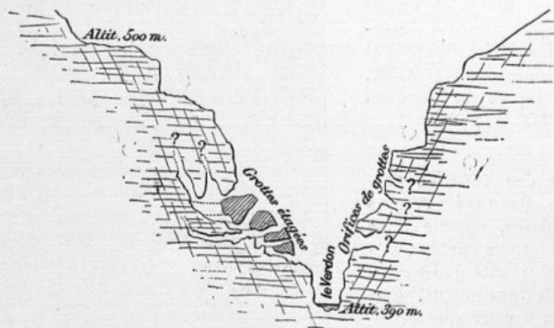
FIG. 41. — Crans de descente d'un cañon et de ses grottes affluentes (Baudinard, Var).
