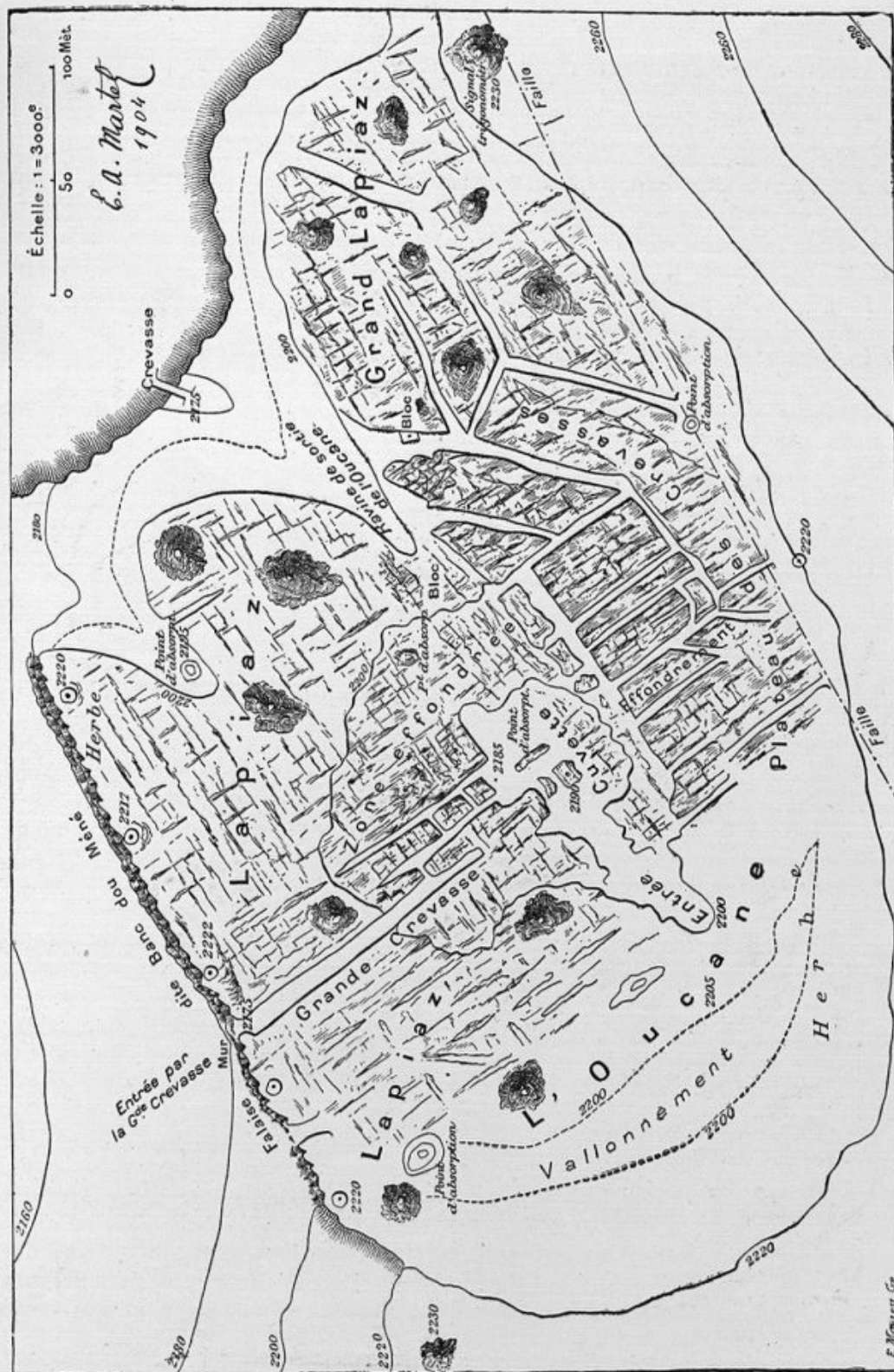
FIG. 38. — Plan du lapiaz de l'Oucane de Chabrières, découvert en 1904 avec MM. David Martin, E. Haug, P. Lory, etc.
