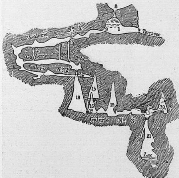
FIG. 26. — Coupe des Baumes-Chaudes (Lozère). (Superposition d'abîmes étagés).
