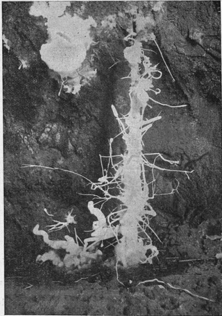
FIG. 28. — Stalagmite ex-centrique.
