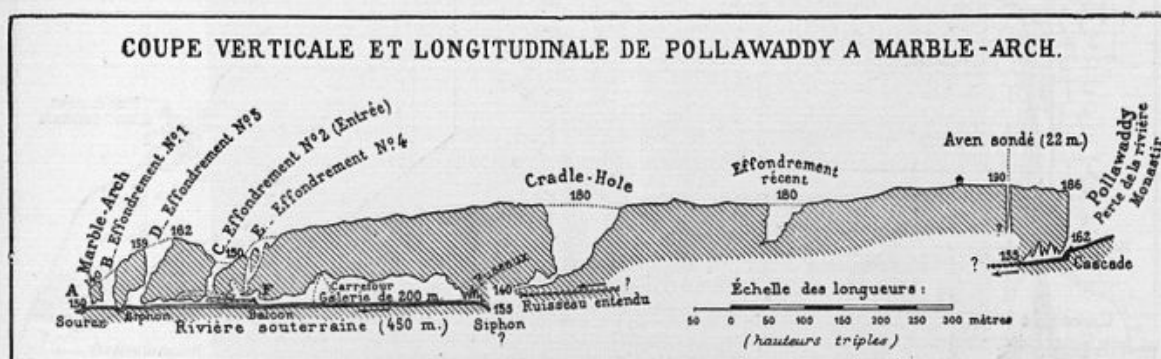
FIG. 2. — Coupe verticale (à Marble-Arch, Irlande) d'un type de circulation souterraine en terrain calcaire : Perte de rivière, — abîmes affluents et regards d'effondrement B ; — grottes, siphons et rivière d'emmagasinement, — résurgence de sortie des eaux A.
