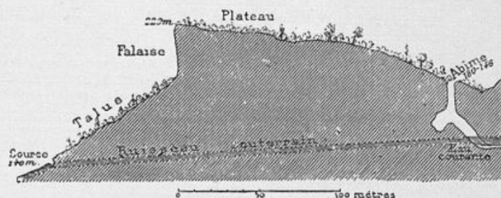
FIG. 22. — Abîme de la Berrie et source de Graudenc (Lot, 1892). Coupe prouvant matériellement la contamination d'une source par un abîme.
