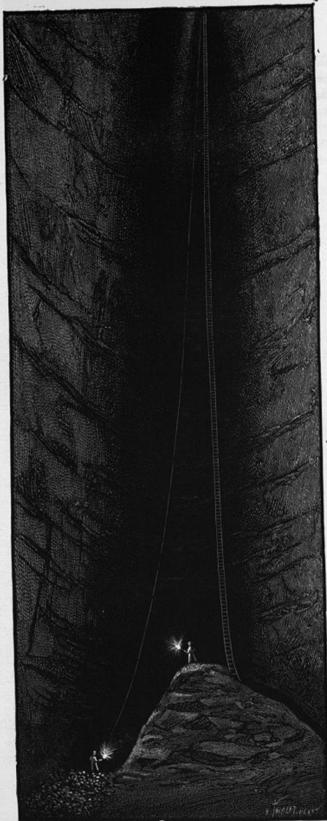
FIG. 27. — Intérieur du gros aven de Canjuers (v. la coupe, p. 39).
