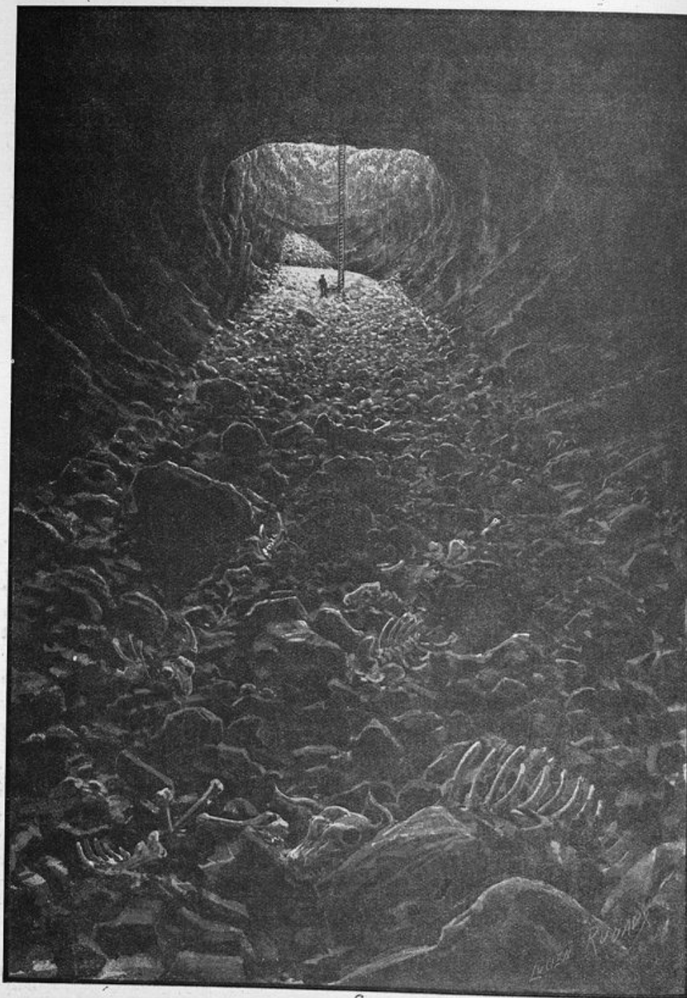
FIG. 23. — Abîme transformé en charnier et contaminant, après les pluies, les eaux souterraines régionales. (Gouffre des Corbeaux, près Bélesta, Ariège : profondeur 110 mètres ; 1907.)
