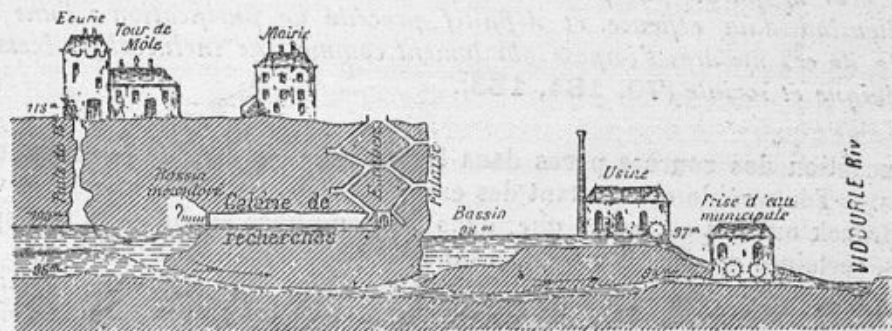
Fig. 24. — Contamination du captage de Saine (Gard) par une écurie (1897) coupe verticale.
