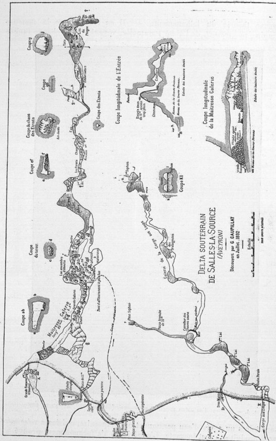
Fig. 5. — Type d'une issue de rivière souterraine disposée en delta (1892-3)
