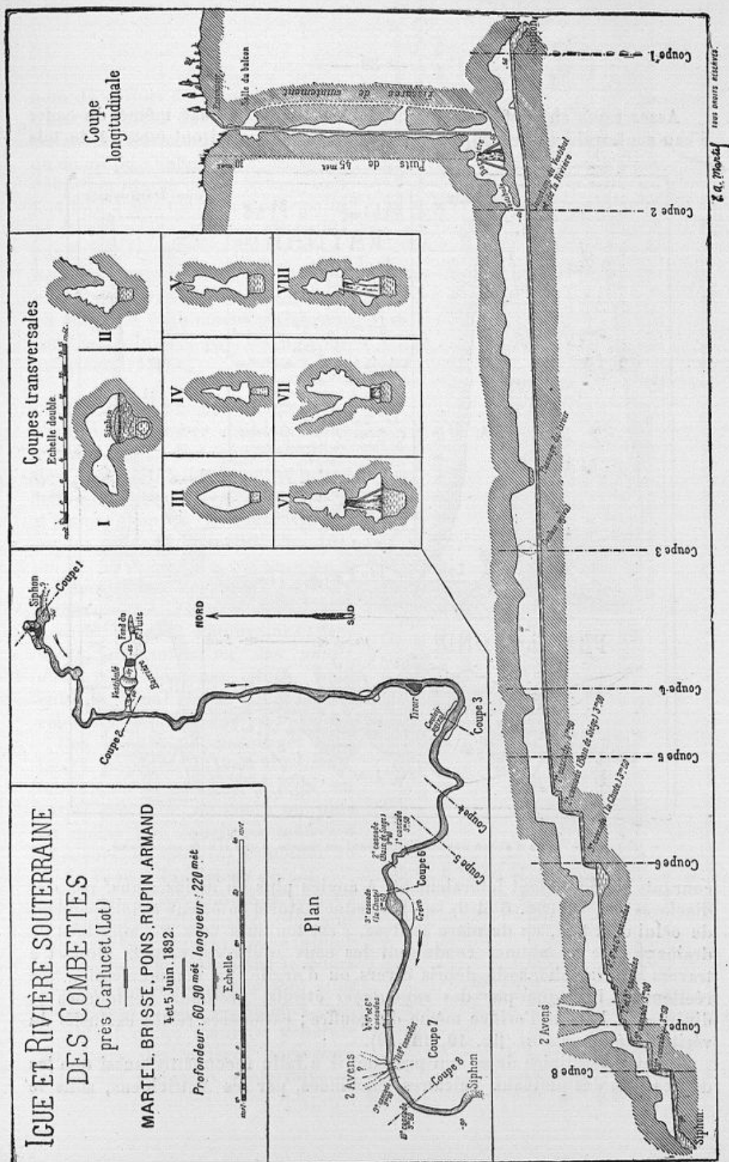
FIG. 6. — Type d'abime greffé indirectement sur une rivière souterraine (1812).
