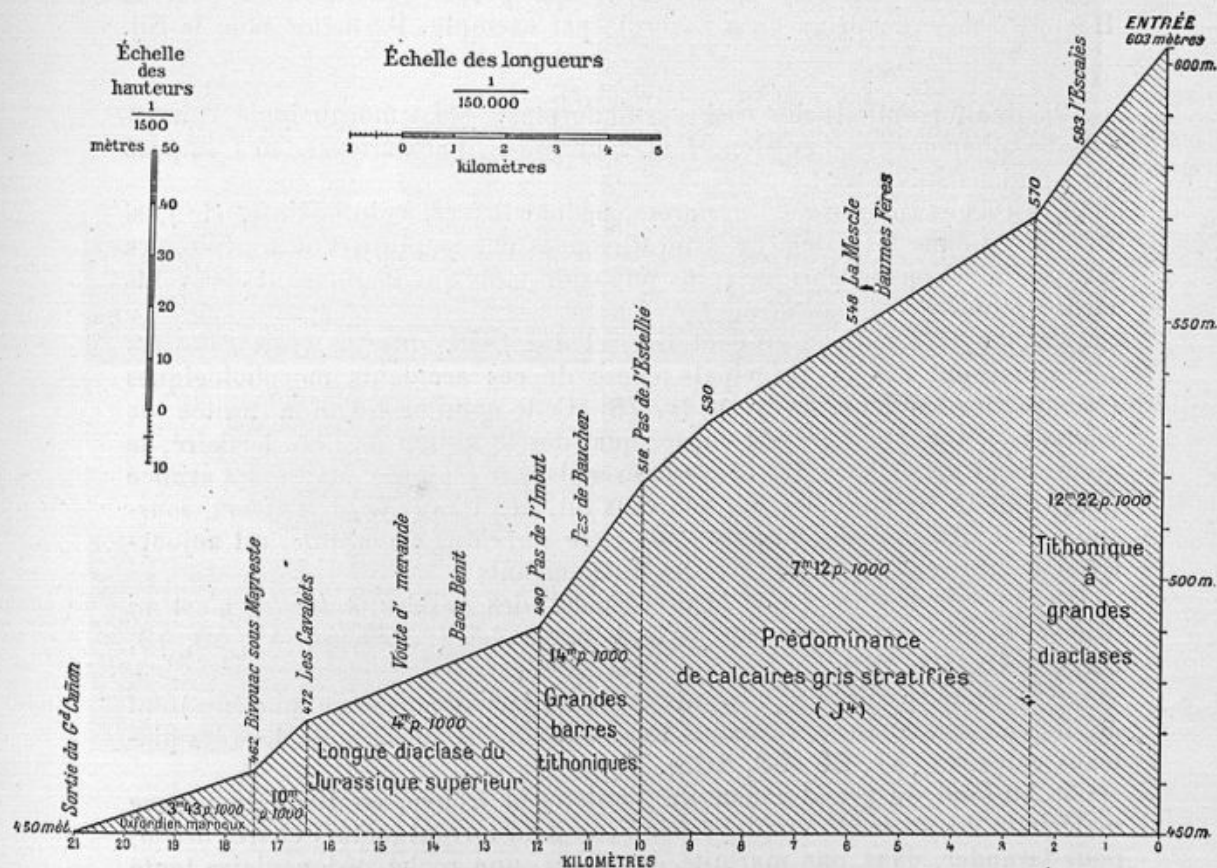
FIG. 35. — Profil en long du Grand Cañon du Verdon (1905-6).
