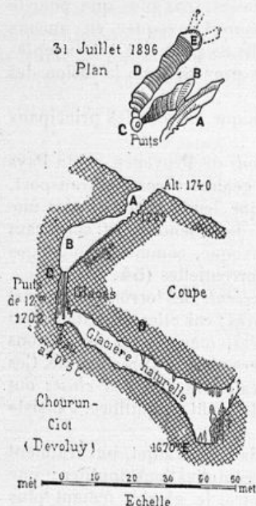
FIG. 42. — Coupe d'un puits à neige en Dévoluy (p. 83).
