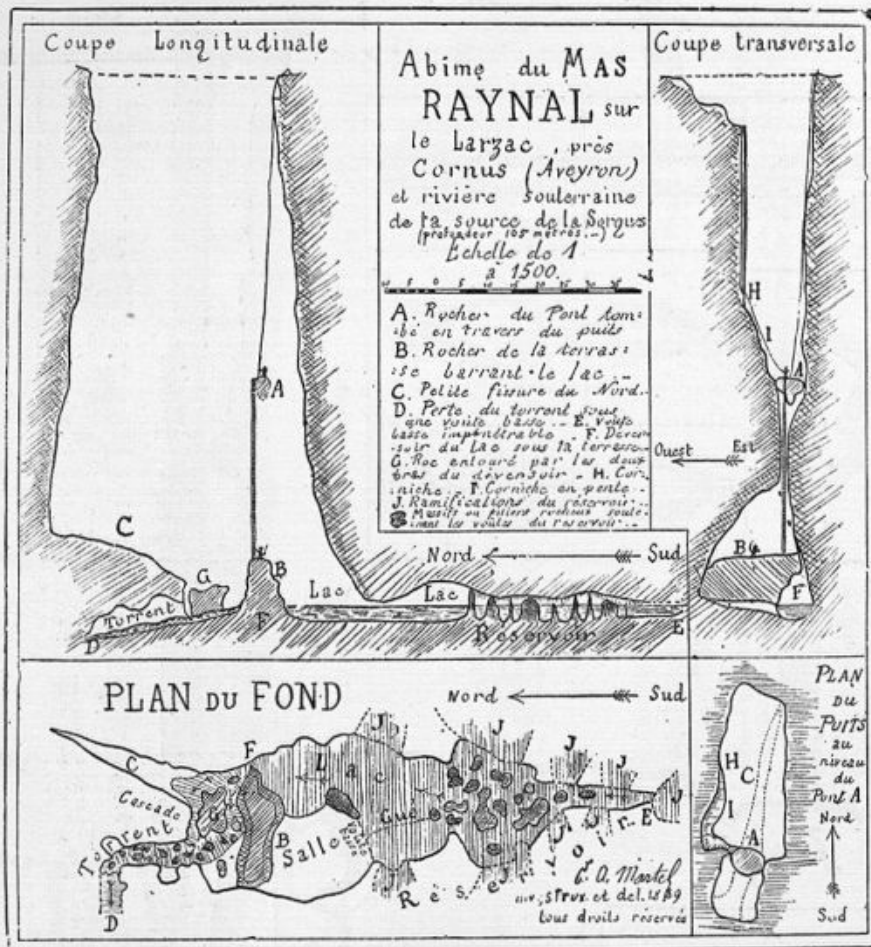
FIG. 7. — Type d'abîme ouvert directement en dessus d'une rivière souterraine.
