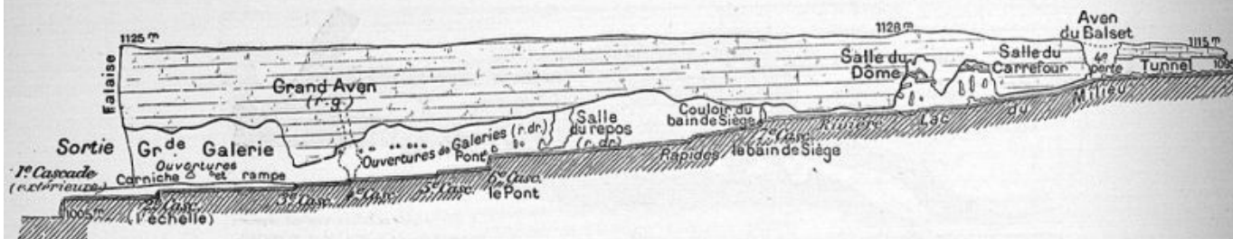
FIG. 16. — Exemple d'une traversée de part en part : Bramabiau, Gard (1888-92).
