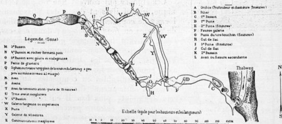
FIG. 13. — Plan d'une source jaillissante (L'Oule, Lot).
