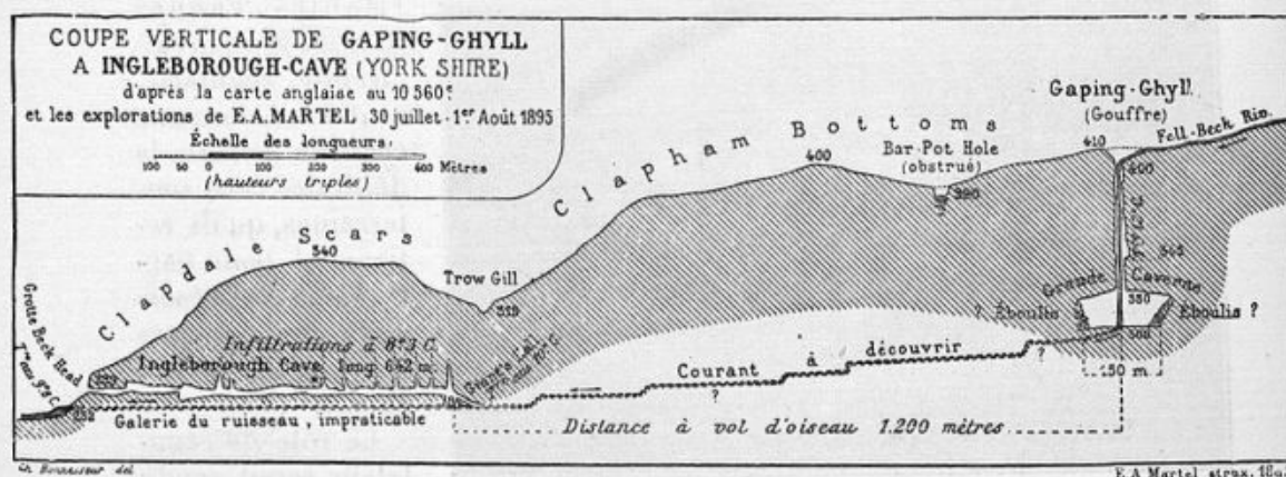
FIG. 17. — Les trois termes de la circulation des eaux souterraines, absorption, emmagasinement. Depuis 1895 de nombreux explorateurs anglais ont révélé tout un réseau de galeries entre le gouffre et l'émergence.
