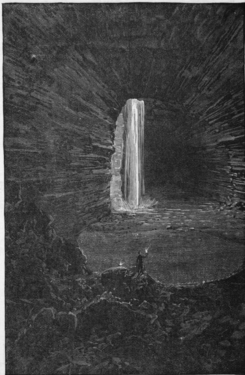
FIG. 4. — Intérieur d'un abîme absorbant et réservoir (Gaping-Ghyll, Angleterre, 1895).
