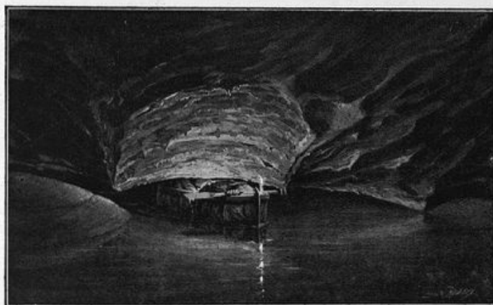
FIG. 15. — Siphon désamorcé; La Bouiche, Ariège (1909).
