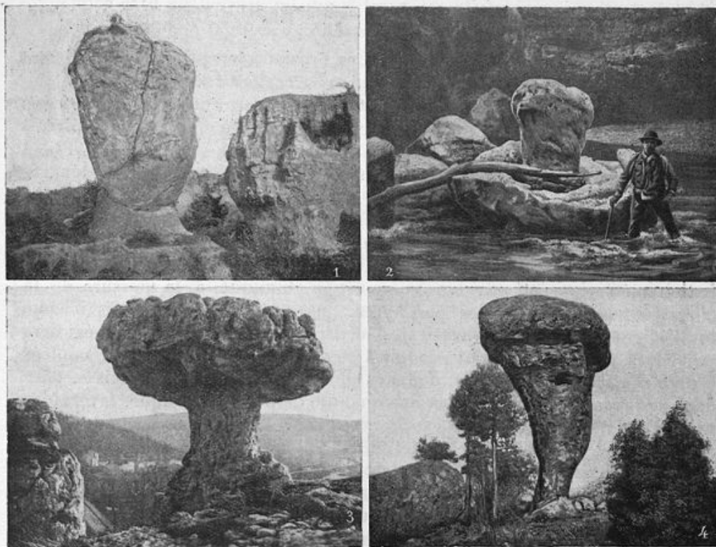
FIG. 36. — Phénomènes anciens et actuel d'érosion torrentielle.
