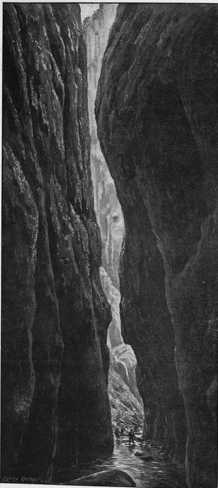
Fig. 44. — Le cañon d'Olhadibre-Holçarté (Basses-Pyrénées, 1908-1909) (V. p. 96). J
