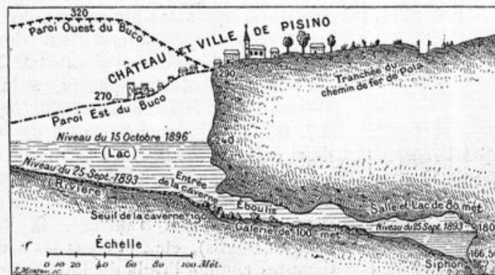
FIG. 12. — Preuve de l'établissement de la pression hydrostatique souterraine, par un siphon, après les pluies. Différence entre les eaux basses et hautes (Foiba de Pisino, Istrie, 1893-1896).
