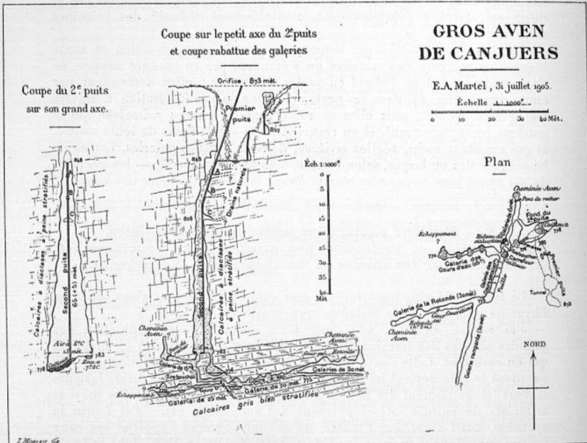
FIG. 21. — Descente des eaux dans un aven : 1 o chute directe dans les diaclasses verticales ; 2 o transformation de la descente en écoulement subhorizontal et en galeries basses et étroites, dans les joints de calcaires très stratifiés.
