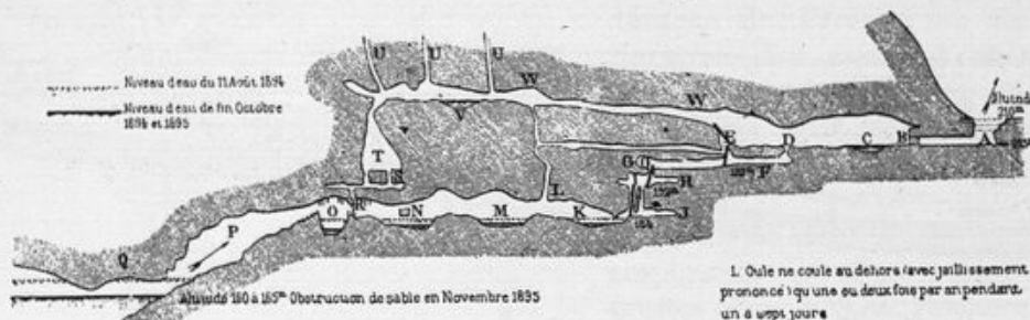
FIG. 14. — Coupe expliquant le mécanisme d'une source jaillissante. Les avens affluents UUU ajoutent leur charge à celle du vase communicant. (V. plan fig. 13).
