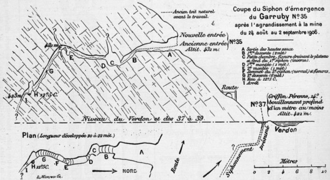
FIG. 34. — Coupe d'un trop-plein de Garruby près Fontaine-l'Evêque (agrandi à la mine en 1906), montrant une paroi de roches qui a résisté à la pression hydrostatique souterraine.
