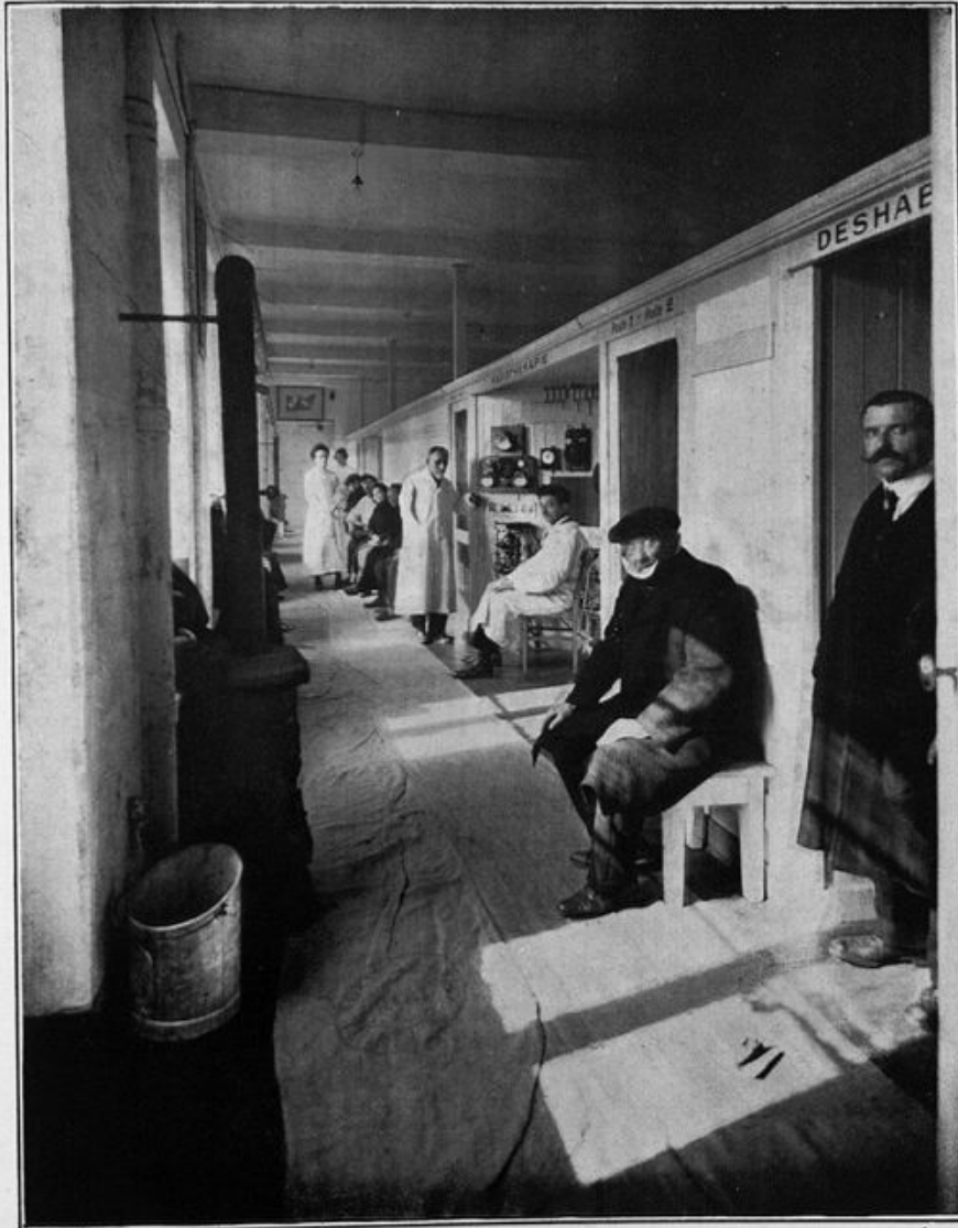
Le couloir servant de salle d'attente aux consultants avec les postes de commande de radiothérapie pénétrante. Plafond et parois de plomb.
