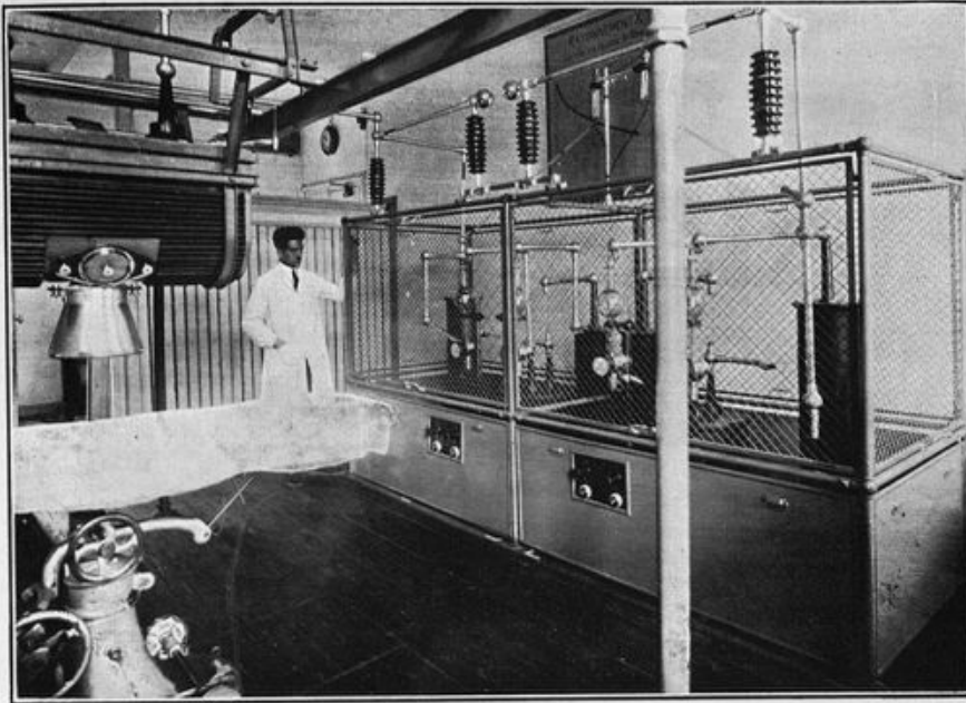
L'appareil de radiothérapie pénétrante à tension constante de Gaiffe, avec parois de protection sur le couloir (5 centimètres de galerie).
