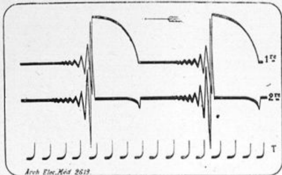
Oscillogrammes d'ondes correctes fournies par un interrupteur bien établi et bien réglé, photographiées avec l'oscillomètre de Blondel.
