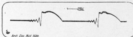
Oscillogrammes du primaire de la bobine avec interrupteur déréglé.
