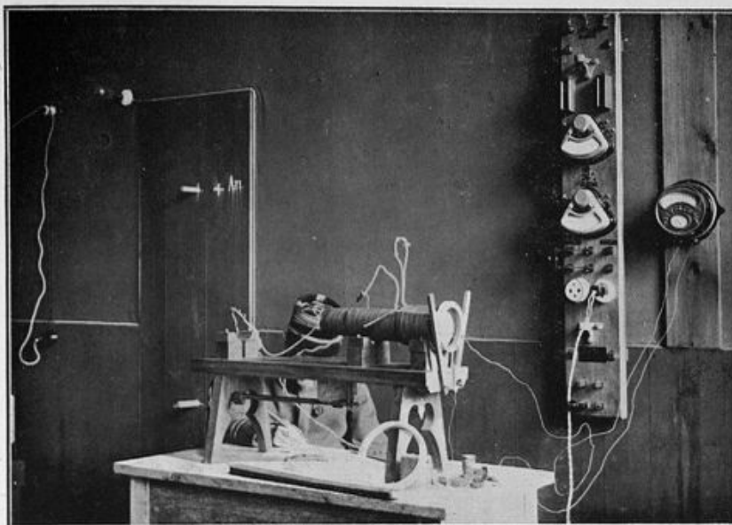
Mesures physiques sur l'électro-vibreur. Intensité apparente. Intensité réelle. Voltage, etc.
