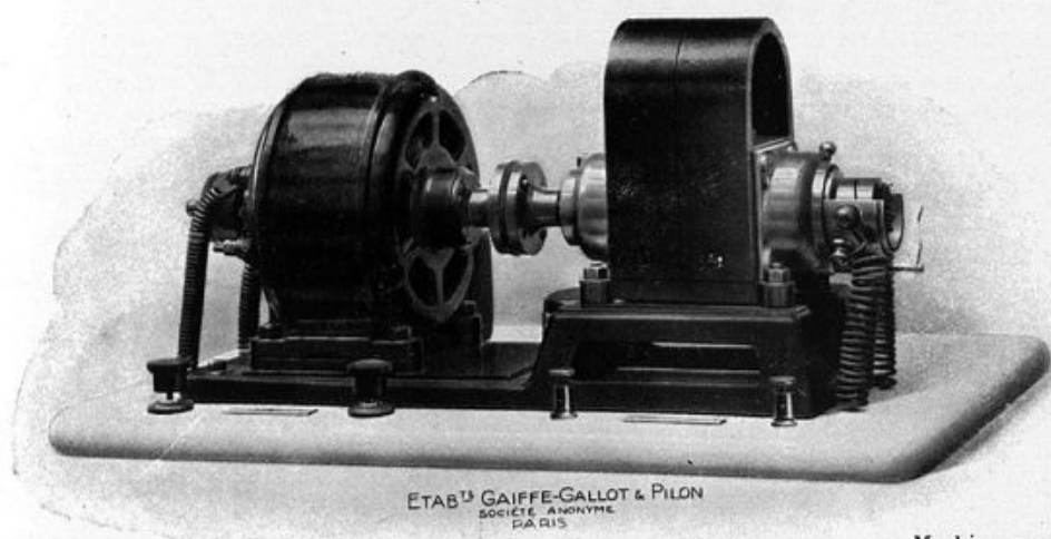
Machine magnéto-faradique.
