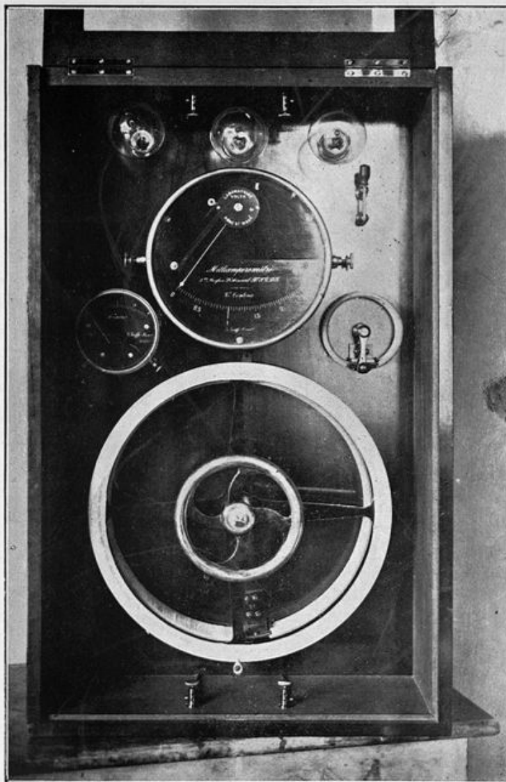
Ohmmètre clinique.
