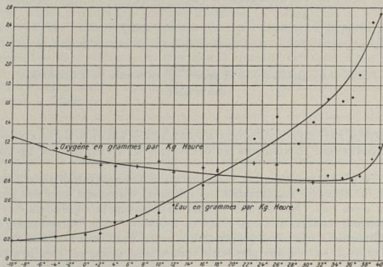
FIG. 26. — Oxygène consommé et eau évaporée par kilog et par heure, par le lapin, en fonction de la température.
