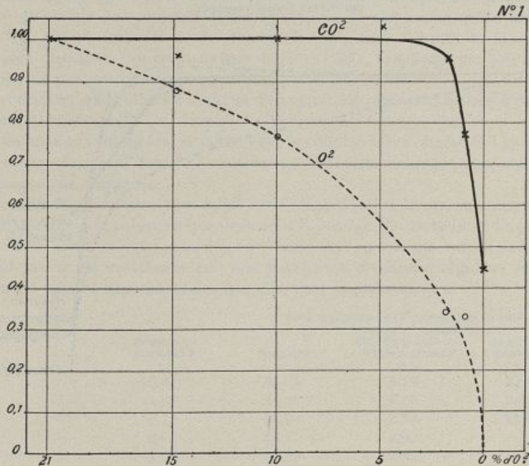
FIG. 10. — Variation des échanges gazeux, chez Hypnum triquetrum , en fonction de la tension d'oxygène de l'atmosphère.
