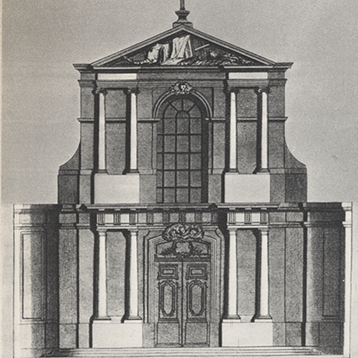
Plan et Elevation du Portail de l'Eglise de la Charité faubourg Saint Germain a Paris Bâti en l'Année 1751. sur les Dessins de Monsieur Cholet Architecte.
