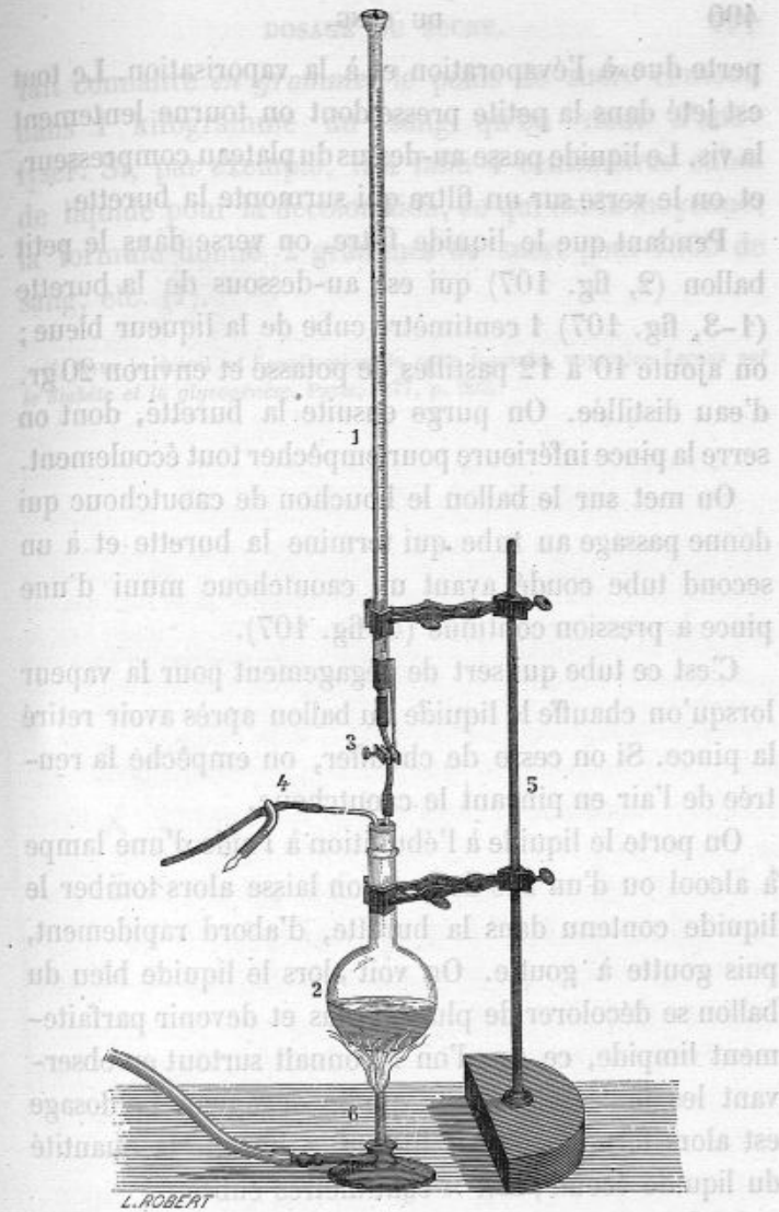
FIG. 407. — Ballon et burette pour le dosage du sucre.
