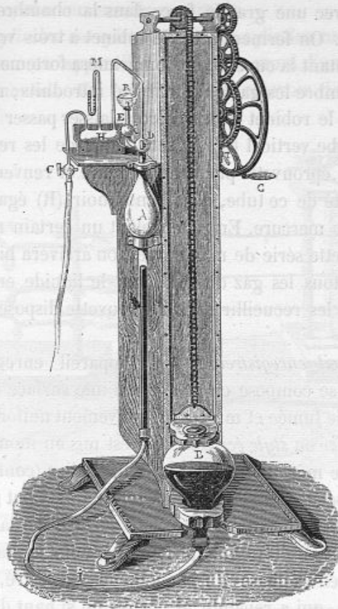
FIG. 66 -- Pompe à mercure.
