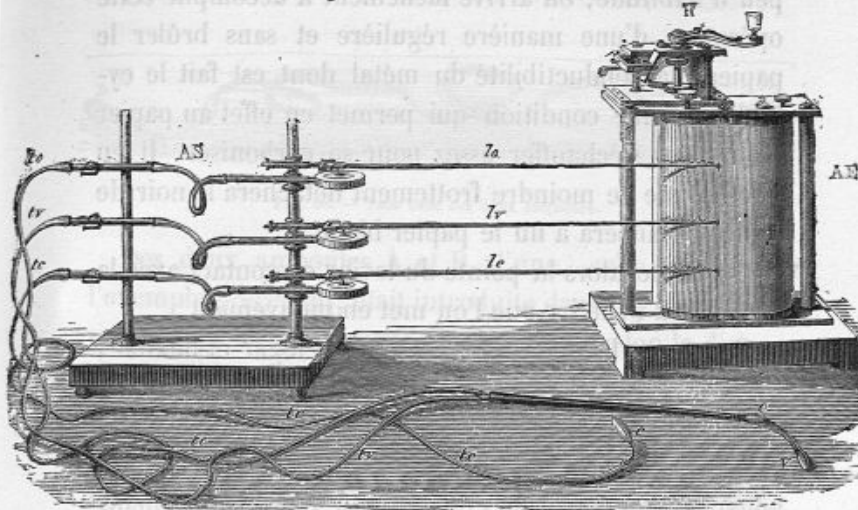
Fig. 67. — Appareil enregistreur.
