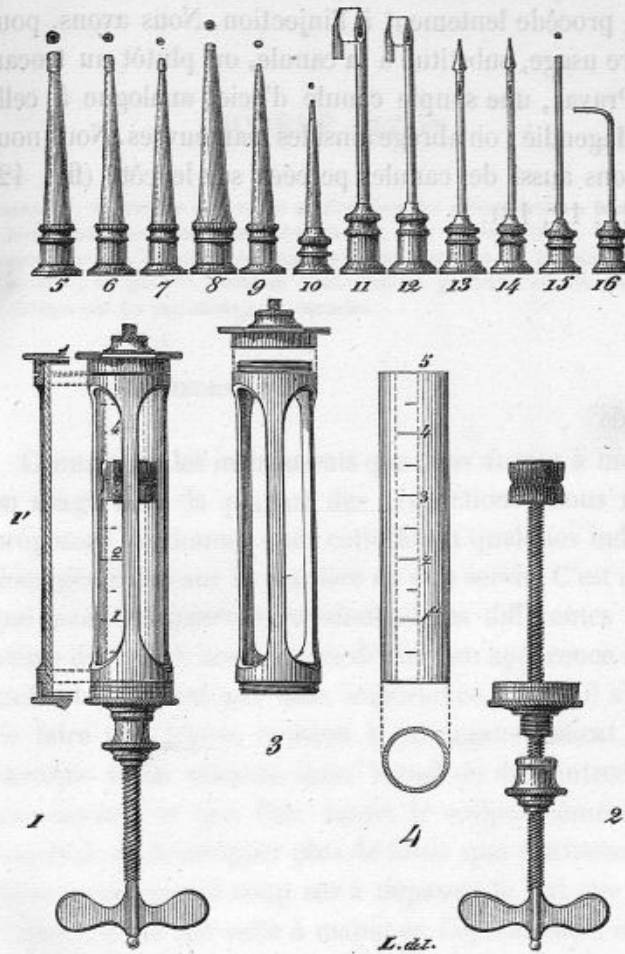
FIG. 42. — Seringue avec ses diverses canules.
