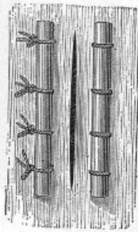
FIG. 54. — Suture enchevillée.
