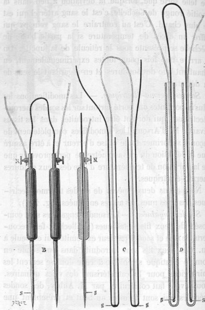
FIG. 101. — Sondes thermo-électriques de d'Arsonval.
