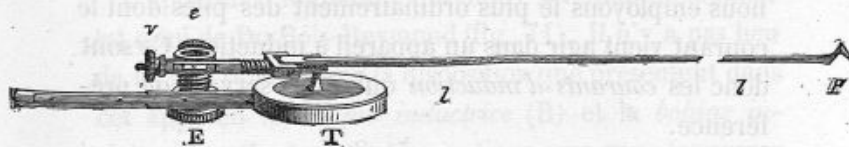
FIG. 69. — Tambour à levier.
