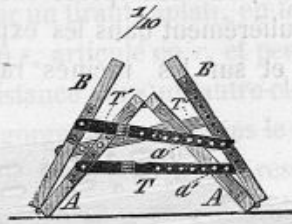
FIG. 18. Table à vivisection en quatrième position : les deux panneaux externes de la figure 17 sont ici rapprochés des panneaux internes, et forment ainsi une étroite gouttière. (Lettres comme dans les figures 10, 15 et 16.)
