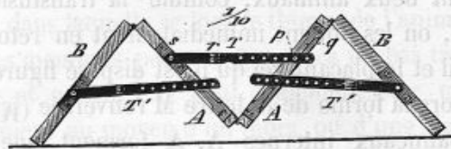
FIG. 16. — Profil de la table à vivisection, dans sa deuxième position (fig. 15), pour montrer les ferrures ou tirants (T, T', T'') avec leurs clous à pivot (s), leurs articulations (r) et leurs clous à tête (p); B, B, panneaux externes; A, A, panneaux internes (formant la gouttière).
