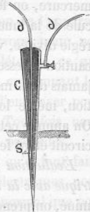
FIG. 402. — Aiguilles.
