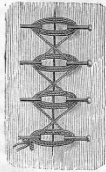
FIG. 51. — Suture entortillée.
