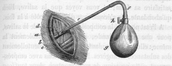
FIG. 112. — Fistule parotidienne chez le cheval, avec canule et petit sac pour recueillir la salive. a , canal de Sténon dans lequel est engagé le tube e ; b , branche du nerf facial; c , artère faciale; f , g , h , détails du robinet et de l'ajutage du petit sac qui reçoit la salive du tube e .
