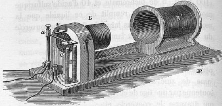
FIG. 71. — Appareil volta-faradique de Du Bois-Reymond.
