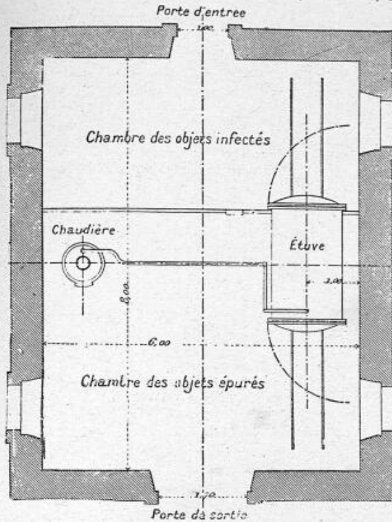
Chambres étuves à désinfection au formol.
