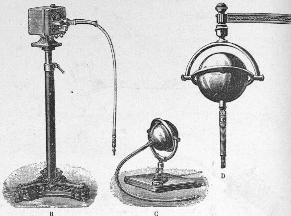
ÉLECTROMOTEURS A COURANT CONTINU AVEC INDUIT EN TAMBOUR MONTÉS AU CHOIX COMME A, B, C, D.
