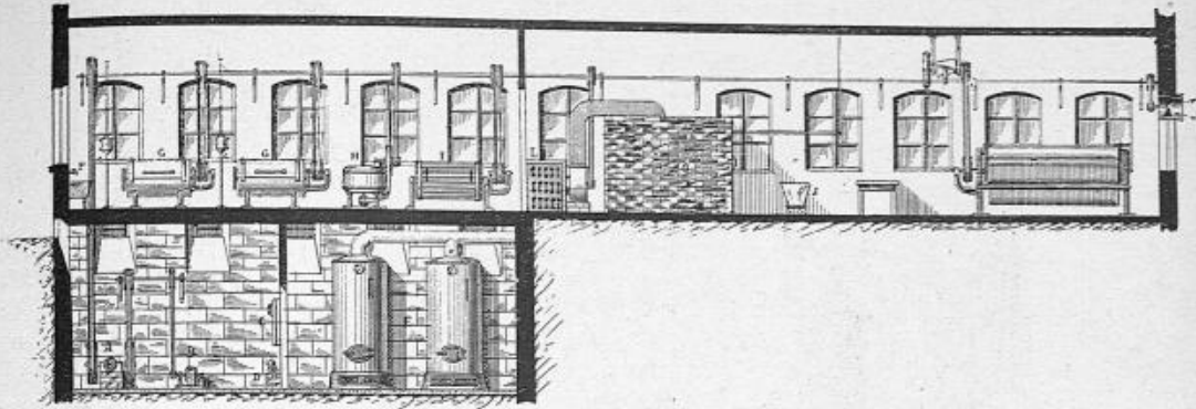
ÉLEVATION LONGITUDINALE.
