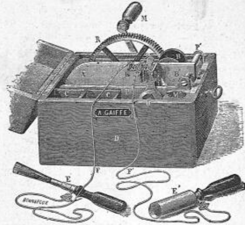
2154: Appareil magnéto-faradique de Gaiffe ..... 60 »
