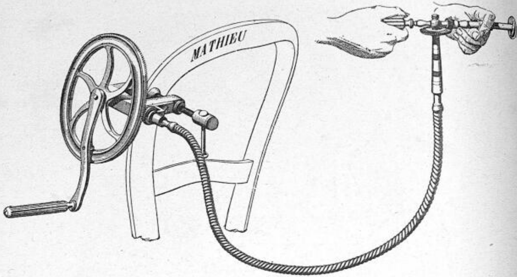
4960, Polytritome de Péan complet en boîte avec 2 couronnes de trépan, 6 forêts, 4 fraises assorties, 4 curseurs gradués, 3 scies et un tire-fond..... 450 »
