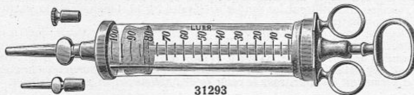
*31293. Seringue argentée du D r Pasteau, capacité 100 cc , corps cristal, soudé au métal, piston caoutchouc stérilisable, pour le lavage du bassin.
