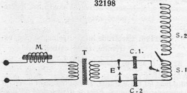
Schéma du montage de d'Arsonval.
