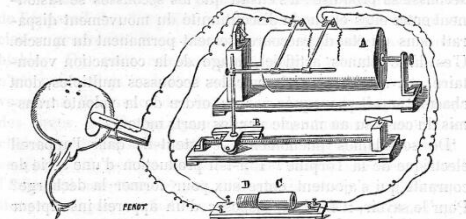
Fig. 1. — Une Torpille est saisie entre les mors d'une pince qui recueille les décharges électriques et les envoie à un signal de Deprez qui les inscrit sur un cylindre; en même temps les décharges traversent la bobine inductrice D. Un autre signal, placé sur le circuit de la bobine induite C, inscrit les courants induits par la décharge.
