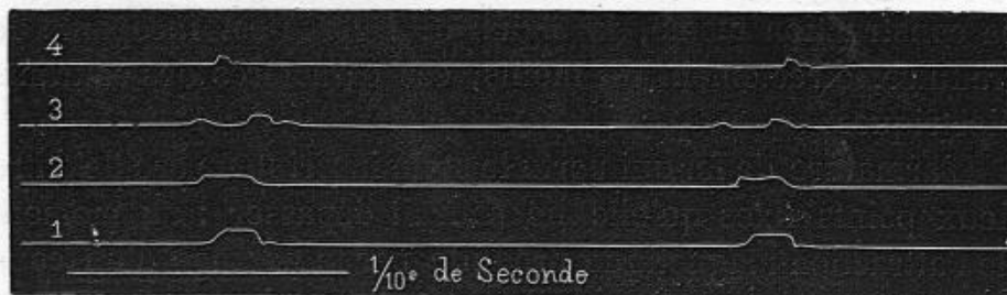
Fig. 13. — Manière dont le signal électro-magnétique traduit des courants électriques de diverses natures.
