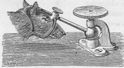
Fig. 139. Appareil contentif pour le rat. Le même modèle sert à fixer la tête du chat.
