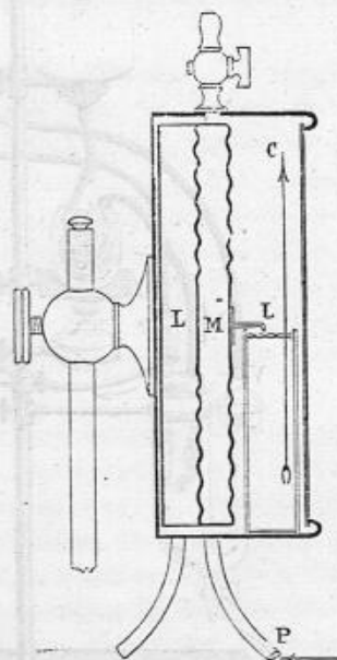
Fig. 150. — Manomètre à cadran et à transmission.
