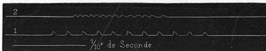
Fig. 6. — Deux tracés de décharge de torpille obtenus avec le signal électrique de M. Deprez.
