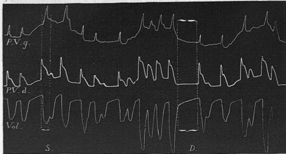
Fig. 116. — Superposition des courbes correspondant aux changements de volume du cœur (ligne Vol), aux pulsations du ventricule droit P.V.d. et du ventricule gauche P.V.g. — On voit chaque systole S, accusée sur les lignes des pulsations P.V.d. — P.V.g. par une ascension de la courbe (durcissement systolique), se traduit sur la ligne des changements de volume (Vol) par un abaissement du tracé (évacuation dans les artères). — La réplétion diastolique D correspond à une forte élévation de la courbe des volumes qui commence au moment du relâchement ventriculaire.
