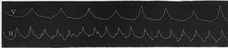
Fig. 126. — Influence du retour à l'horizontale (ligne H) sur le rythme cardiaque et respiratoire d'un lapin placé en attitude verticale (ligne V). — Mouvement du cylindre enregistreur considérablement ralenti.
