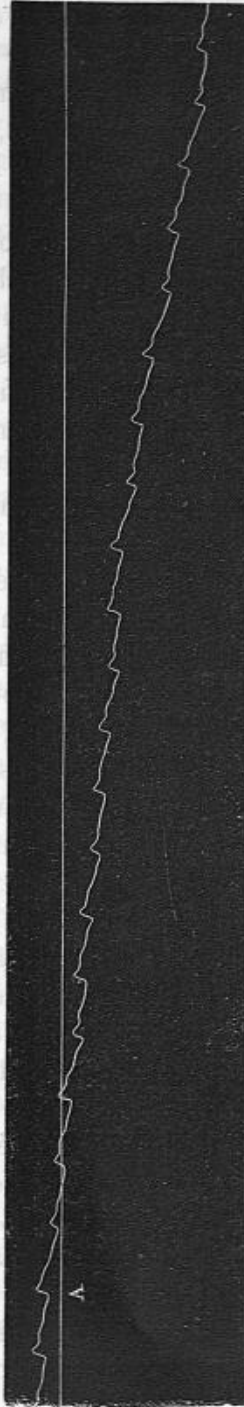
Fig. 80. — Diminution rapide et considérable du volume de la main produite par l'aspiration d'une grande quantité de sang vers le membre inférieur enfermé dans la ventouse de Junod.
