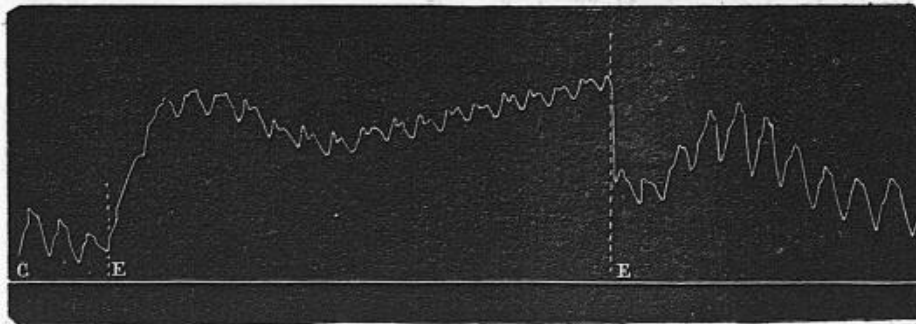
Fig. 73. — Augmentation du volume du cerveau pendant l'effort de E sur E. Pulsations plus fréquentes et dicotes.
