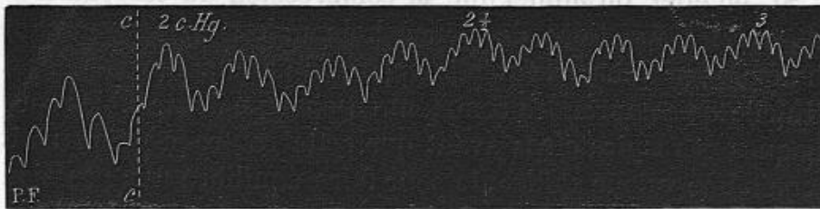
Fig. 134. — Exemple d'accélération des battements du cœur, survenue dans une expérience de compression cérébrale, entre 2 et 3 \frac{1}{2} c. Hg. La pression fémorale (PF) dont ce tracé donne les variations, s'élève en même temps que le cœur s'accélère : ce double effet paraît dû aux efforts de l'animal.
