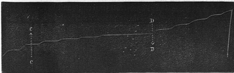
Fig. 61. — Ondées sanguines fournies par un cœur de tortue soumis à une circulation artificielle. Ces ondées diminuent à partir du début de la contre-pression exercée sur le cœur (en CC) ; elles se suppriment complètement à partir d'un certain degré de compression, et reparaissent quand on décomprime, en DD.
