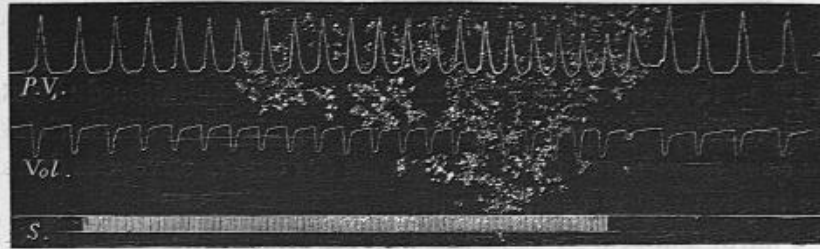
Fig. 109.— Changements de volume (Vol.) et pulsations du cœur (P V) pendant l'excitation de la première branche accélératrice. La fréquence et la durée des excitations sont indiquées par le signal électro-magnétique (ligne S).
