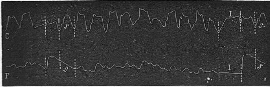
Fig. 46. — P. Pouls radial. — C. Pulsations du cœur. — On voit en ss deux systoles sans pulsation artérielle correspondante ; en I , une intermission vraie du cœur. (Hop. Necker, service du Prof. Potain, 16 juillet 1876). — (Insuffisance mitrale.)
