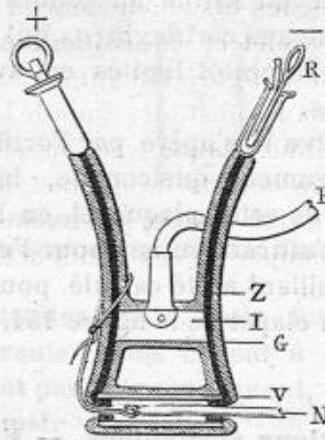
Fig. 457. Excitateur isolé. — P, tige en plomb fixée à une plaque d'ivoire I ; Z, tige de zinc amalgamé formant conducteur ; V, tube de verre isolant les deux zincs ; G, gutta-percha isolant l'appareil ; N, nerf introduit dans le tube excitateur et fixé avec un fil. (Le fil doit toujours être introduit par le plus petit orifice avant la ligature du nerf : c'est par le glissement de ce fil dans l'anneau qu'on attire le nerf dans le tube).
