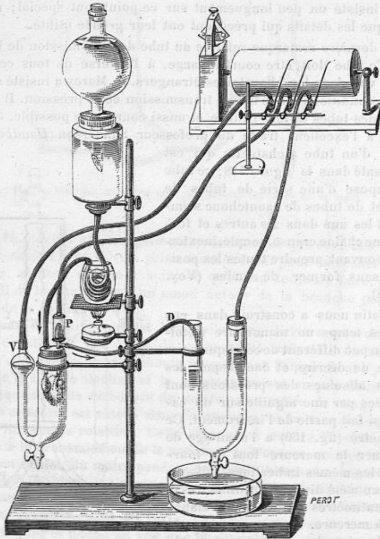
Fig. 154. Appareil à circulation artificielle pour le cœur de la tortue, permettant d'étudier les changements de volume du cœur (v), les variations de la pression artérielle (p) et les débits (b) correspondant aux systoles. — (Les hauteurs des niveaux du sang dans le tube en U où se fait l'écoulement D doivent être interverties.)
