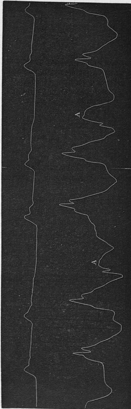
Fig. 47. — Puls bigéminé et cœur sur le Schéma. — Tracés simultanés de la carotide et de la pulsation cardiaque. — Le pouls carotidien (ligne supérieure) présente des avortements périodiques. — Le tracé de la pulsation ventriculaire présente, en correspondance avec les pulsations carotidiennes avortées, des courbes plus basses que de coutume et caractéristiques de l'insuffisance mitrale.
