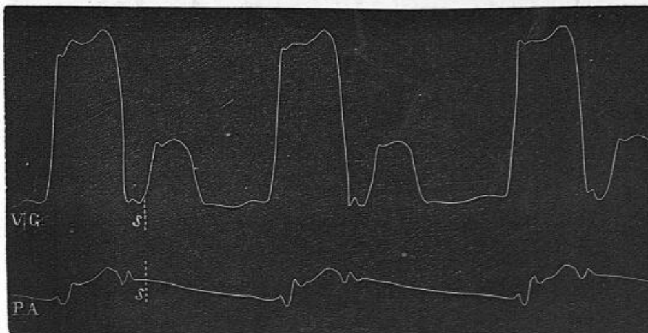
Fig. 37.— V.G, Pression ventriculaire gauche. — P.A, Pression aortique. — Deux systoles du cœur pour une pulsation artérielle ; s, systole avortée. ( Expériences inédites , Chauveau et Marey ; Lyon, 19 novembre 1862.)
