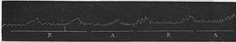
F g. 42. — Pulsations du cœur d'un lapin profondément chloralisé. — Phases d'accélération AA. — Ralentissement des pulsations pendant les phases RR.
