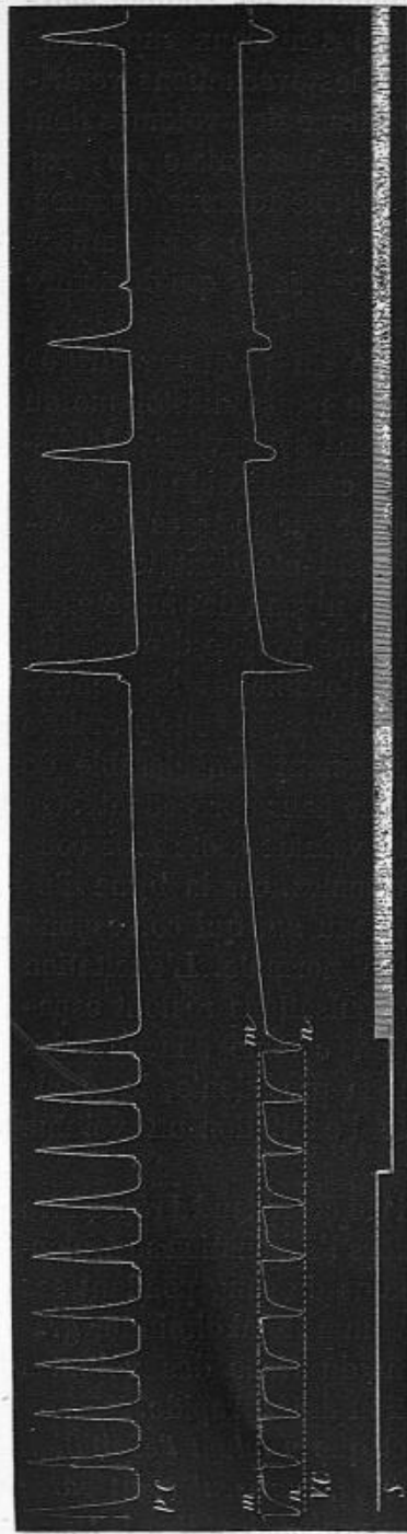
Fig. 410. — Pulsations du cœur (P. C.) et changements de volume (V. C.) Avant l'excitation du bout périphérique du pneumogastrique droit, on voit que tous les changements diastoliques et systoliques de volume s'opèrent entre les deux lignes de niveau mm , nn . Pendant l'excitation indiquée par le signal S , le volume du cœur augmente graduellement et les évacuations et les évacuations sont moins profondes.
