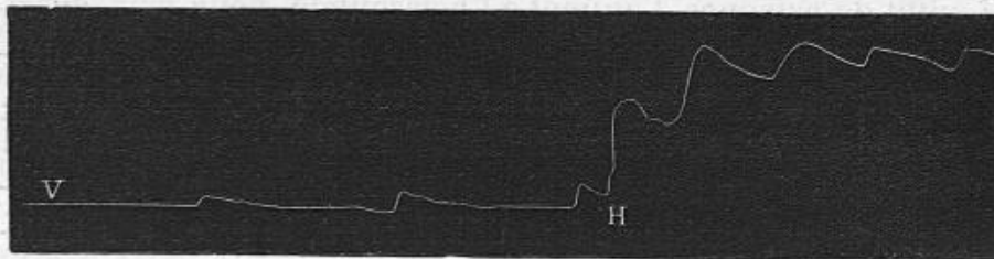
Fig. 127. — Respiration d'un lapin sur le point de succomber dans la position verticale (V); le retour à l'horizontale (H) rend aussitôt sa respiration plus fréquente et plus ample.
