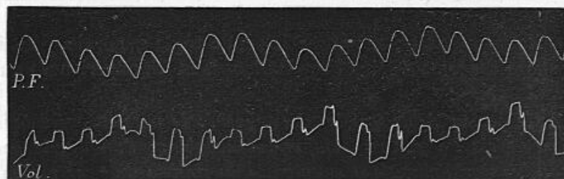
Fig. 401. — Changements de volume du cœur (ligne Vol) et variations de la pression fémorale (P F).
