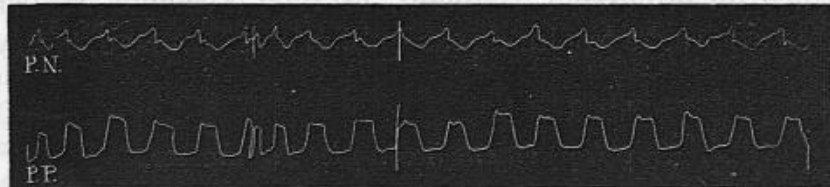
Fig. 146. P.N. Pulsations négatives , et pulsations positives P, P recueillies simultanément. Opposition des courbes des changements de volume P N et des changements de consistance P P.
