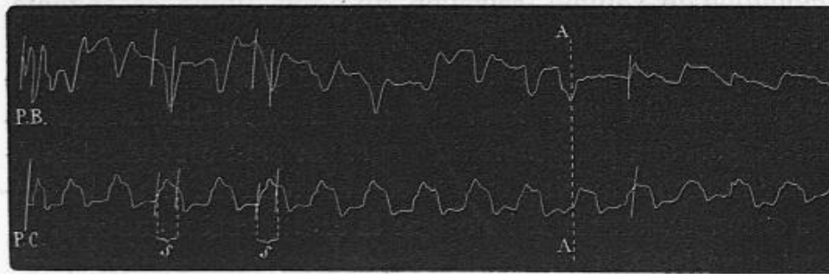
Fig. 120. — P.B., variations de la pression buccale exprimant les changements de volume du cœur.—P.C., pulsations du cœur.—S, systoles. Pulsations des artères bucco-pharyngiennes quand la glotte est fermée, à partir de AA.
