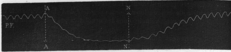
Fig. 62.— Comparaison des effets produits par la compression des veines caves en AA' sur la pression fémorale (PF) et des résultats de la contre-pression exercée sur le cœur. En NN, on rétablit le cours du sang veineux.
