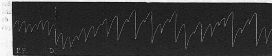
Fig. 136. — Ralentissement du cœur produit par la décompression brusque du cerveau faite en D. (Tracé des variations de la pression fémorale.)
