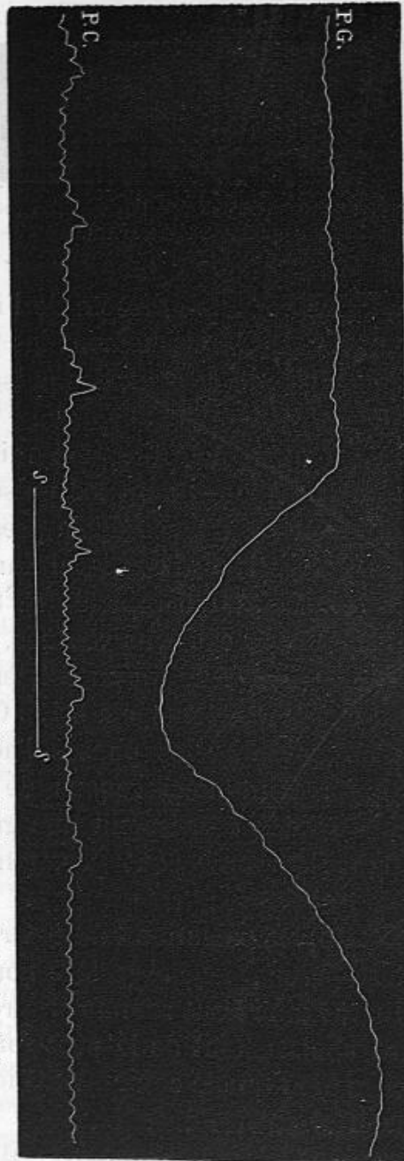
Fig. 43. — Pulsations du cœur (P. C.) et variations de la pression carotidienne (P. G.) sur un lapin chloralisé; abaissement de pression et disparition des pulsations artérielles pendant une phase de systoles avortées ss.
