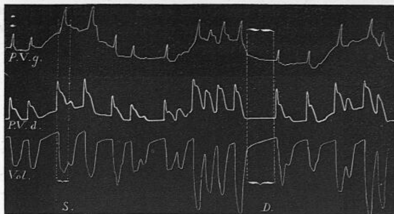
Fig. 400. — Superposition des courbes correspondant aux changements de volume du cœur (ligne V), aux pulsations du ventricule droit V D et du ventricule gauche VG. — On voit chaque systole S, accusée sur les lignes des pulsations PD — PC par une ascension de la courbe (durcissement systolique), se traduire sur la ligne des changements de volume VC par un abaissement du tracé (évacuation dans les artères). — La réplétion diastolique D correspond à une forte élévation de la courbe des volumes qui commence au début même du relâchement ventriculaire.
