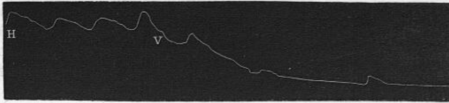
Fig. 128. — Respiration d'un lapin dont l'attitude horizontale avait rétabli la régularité respiratoire (H). Le retour à la verticale (V) abolit presque complètement la respiration.
