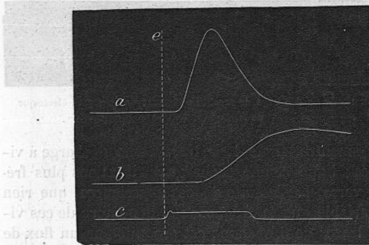
Fig. 7. — Comparaison du retard des signaux fournis par le muscle de Grenouille avec l'instantanéité du signal électro-magnétique.
