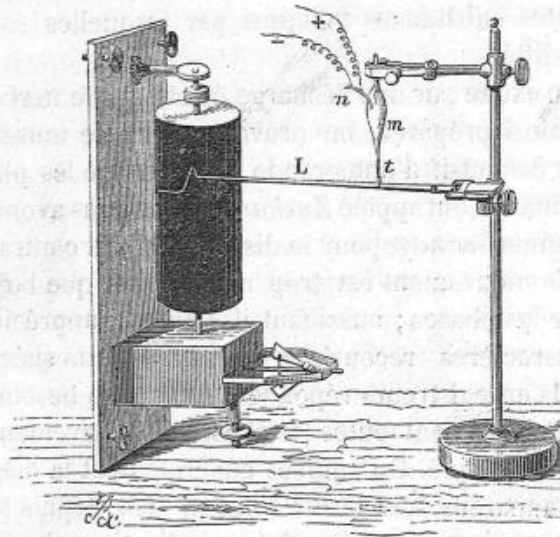
Fig. 2. — Description théorique du myographe.
