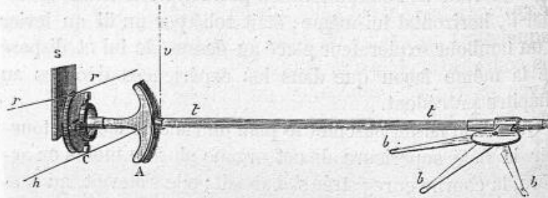
Fig. 109. — Disposition réelle de l'appareil explorateur des mouvements de l'aile et de ses changements de plan.
