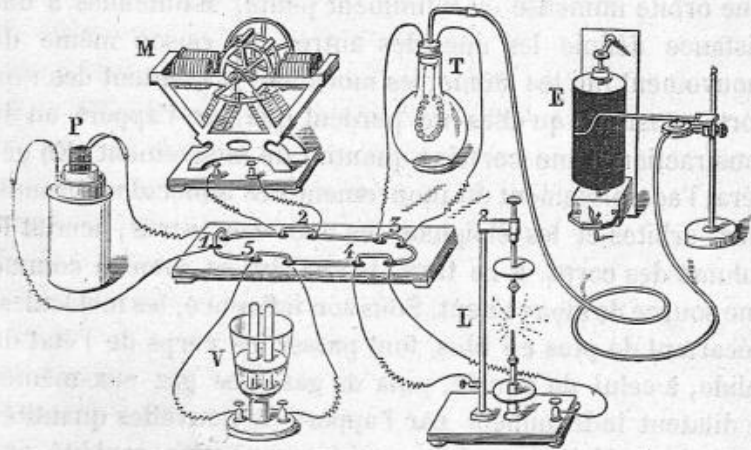
Fig. 1. — Montrant la transformation de l'électricité d'une pile, en travail mécanique, en chaleur, en lumière et en action chimique.
