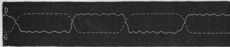
Fig. 25. — D Tracé des appuis et levés du pied droit fournis par un levier soumis en même temps à 10 vibrations par seconde. On voit que les vibrations occupent plus de longueur à la fin de l'appui du pied, cela exprime la plus grande vitesse de translation du corps à ce moment. — La même accélération s'observe à la fin de la période de soutien du pied droit; elle s'explique par l'action du pied gauche qui est, à ce moment, à la fin de son appui.
