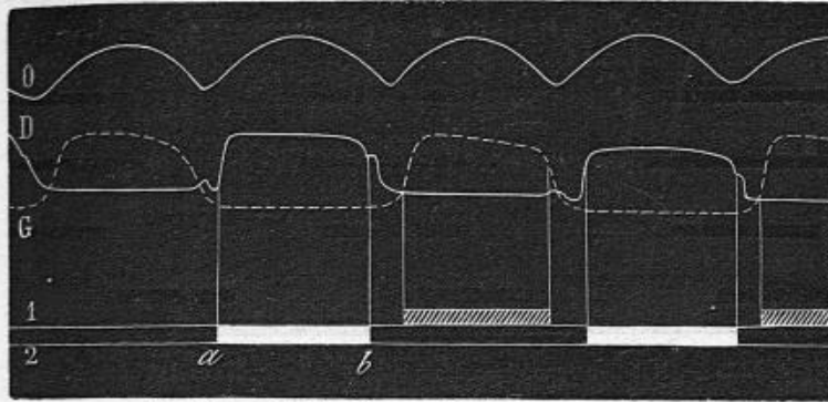
Fig. 34. — Notation d'un tracé de la course de l'homme.
