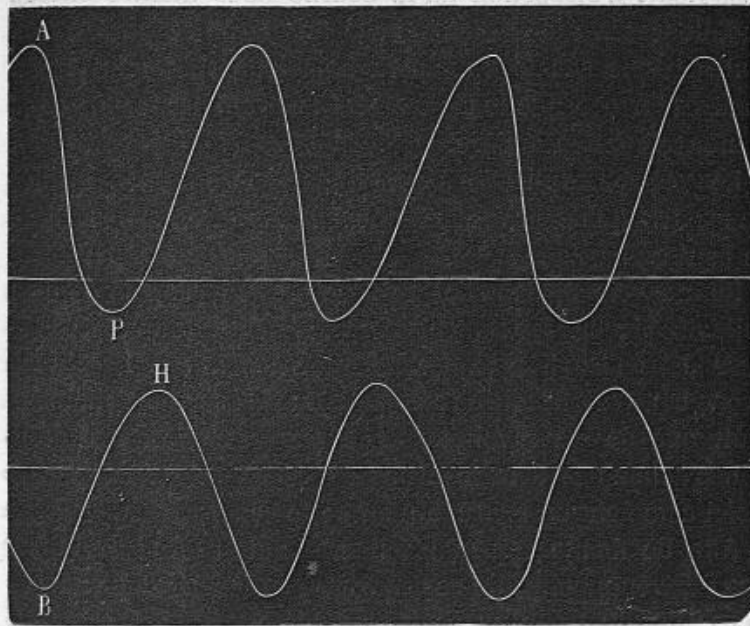
Fig. 105. — Tracés des mouvements de l'aile du pigeon. — Ligne supérieure AP mouvements d'ayant en arrière. Ligne inférieure HB mouvements de haut en bas.
