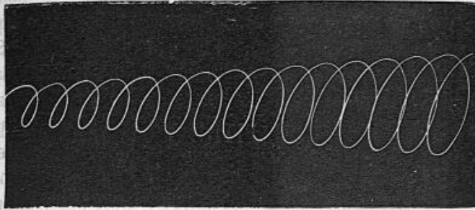
Fig. 101. — Parcours elliptique de la pointe de l'aile d'un oiseau.
