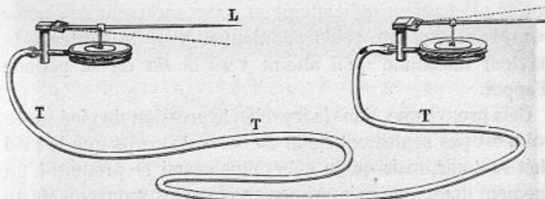
Fig. 21. — Transmission d'un mouvement d'oscillation à l'appareil enregistreur.
