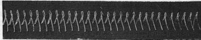
Fig. 79. — Graphique d'une verge de Wheatstone accordée à l'octave, munie d'une aile de guêpe et orientée de manière à enregistrer surtout la boucle supérieure du 8.
