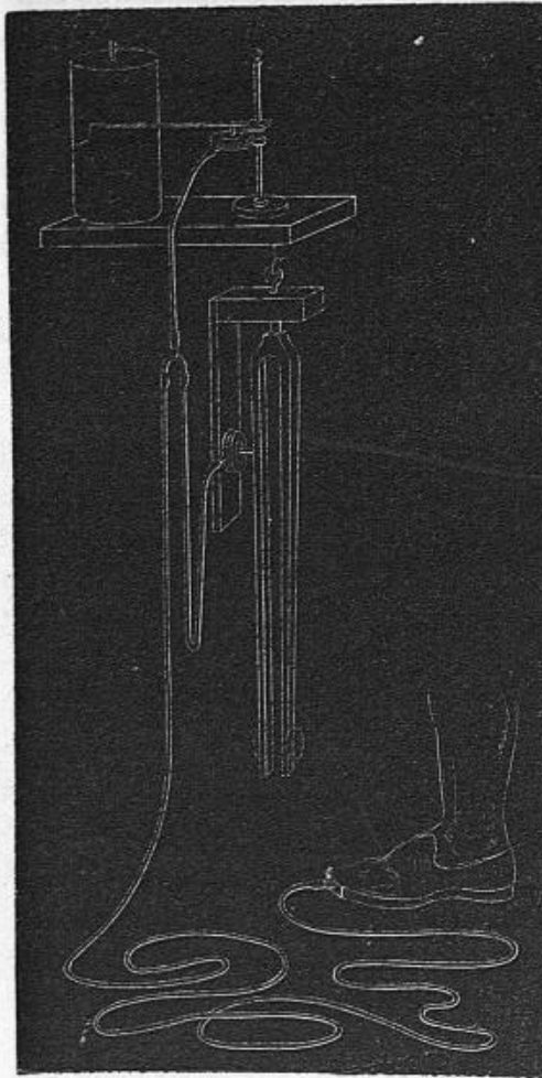
Fig. 26. — Un gros diapason dont les vibrations sont réduites par des masses de plomb à 10 par seconde agit, par un tambour explorateur relié à l'une de ses branches, sur le tambour à levier enregistreur. Celui-ci reçoit en même temps, par un tube bifurqué, l'influence des appuis et des levés des pieds du marcheur.
