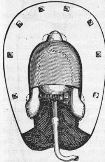
Fig. 42. — Appareil explorateur de la pression du sabot du cheval sur le sol.
