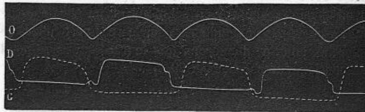
Fig. 30. — Tracé de la course de l'homme. — D (courbe formée d'un trait plein), appuis et levés du pied droit. — G (courbe ponctuée) action du pied gauche. — O oscillations ou réactions verticales du corps.
