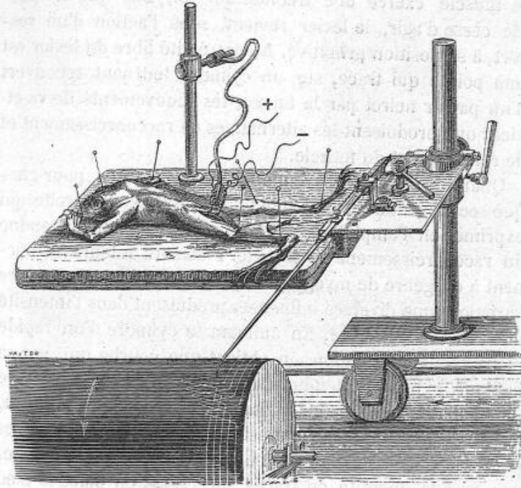
Fig. 3. — Myographe de Marey.
