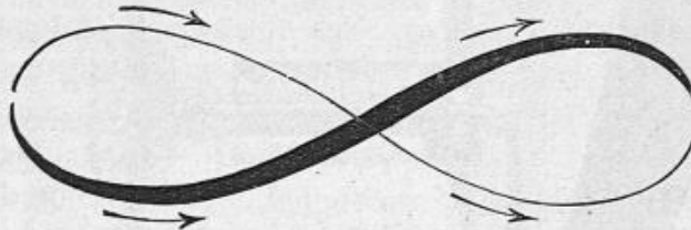
Fig. 86. — Trajectoire de l'aile.
