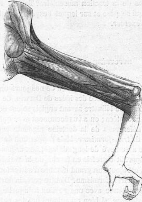
Fig. 18. — Muscles de la cuisse chez le Coaita . — Droit interne, s'insérant loin du genou, presque entièrement dépourvu de tendon. — Le conturier ayant son attache supérieure, très-éloignée de l'articulation coxo-fémorale, a des mouvements très-étendus; il possède en conséquence une grande longueur de fibre rouge et pas de tendon.
