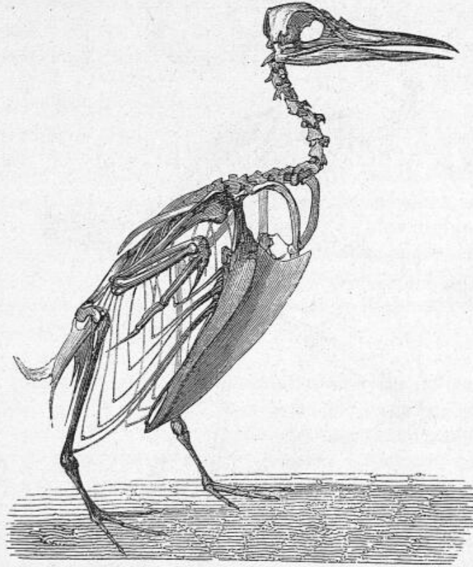
Fig. 14. — Squelette d'un pingouin ; sternum très-long, aile très-courte.
