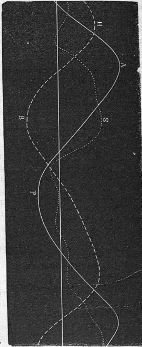
Fig. 110. — Traçé simultané des divers mouvements de l'aile d'une buse. — La courbe AP indique les mouvements de l'aile en avant et en arrière. — HB exprime le mouvement de haut en bas. — La courbe ponctuée indique la torsion de l'aile autour de l'articulation scapulo-humérale; plus la courbe s'élève au-dessus de l'axe des abscisses, plus elle exprime que le bord postérieur de l'aile est relevé.
