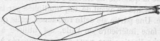
Fig. 116. — Aile d'un Insecte.
