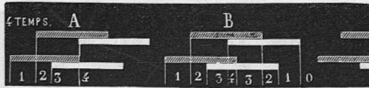
Fig. 62. — Notation du galop à quatre temps. A, détermination de chacun des temps successifs. B, détermination du nombre des pieds qui supportent le corps à chaque instant.
