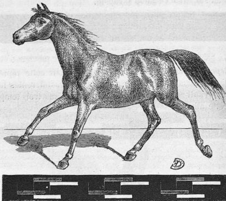
Fig. 60. — Cheval au 3 e temps du galop à droite.
