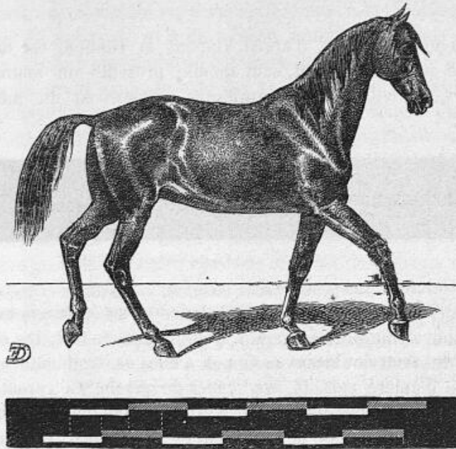
Fig. 34. — Représentation du cheval au pas.
