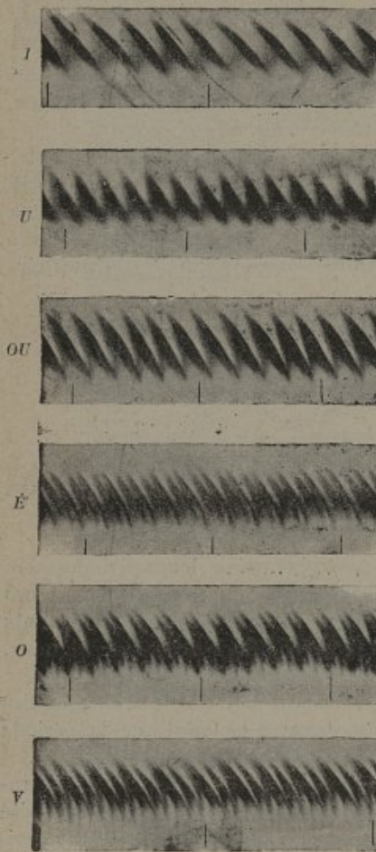
FIG. 15. — Flammes manométriques obtenues sans embouchure par M. Marage.
