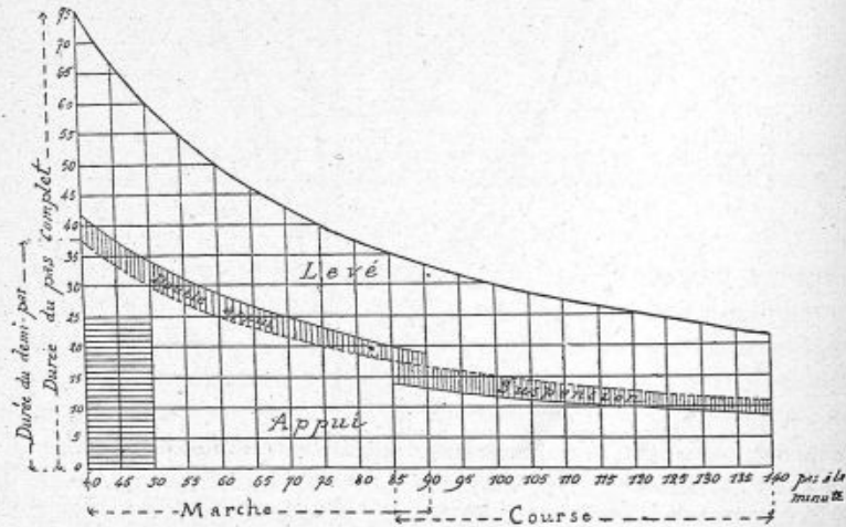
Fig. 364. — Comparaison de la durée de l'appui et du lever du pied, du double appui et de la suspension dans la marche et la course (DEMÉNY).
