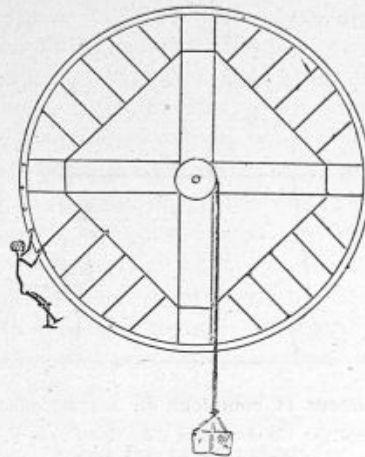
Fig. 561. — Manière défectueuse d'utiliser la force musculaire de l'homme sur un treuil en grim pant à la force des bras.
