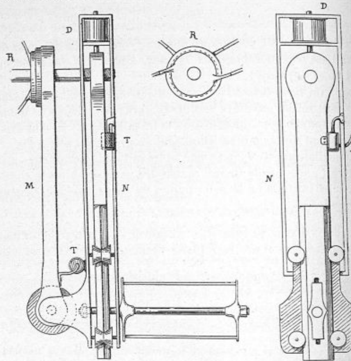
Fig. 554. — Manivelle dynamographique pour mesurer le travail dans le vélocipède (DEMÉNY).
