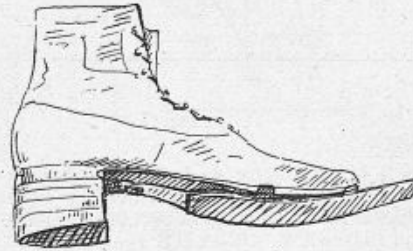
Fig. 318. — Chaussure destinée à faire des expériences sur l'influence de la hauteur du talon et de la longueur de la semelle sur la longueur du pas.
