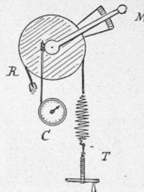
Fig. 563. — Manivelle dynamométrique donnant l'indication de la force motrice nécessaire à vaincre le frottement sous la tension du ressort TR agissant sur un tambour. Un compteur C donne la mesure du chemin parcouru par la manivelle ce qui permet d'évaluer le travail produit.
