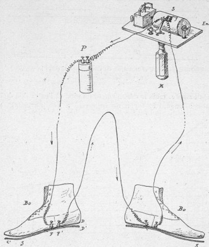
Fig. 309. — Dispositif pour mesurer la durée du double appui dans la marche (DEMENTY).
