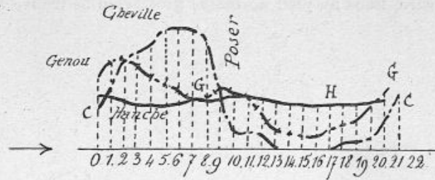
Fig. 302. — Variations de la vitesse horizontale de la hanche, du genou et de la cheville pendant un pas complet de marche; les temps sont comptés en 20 e de seconde.
