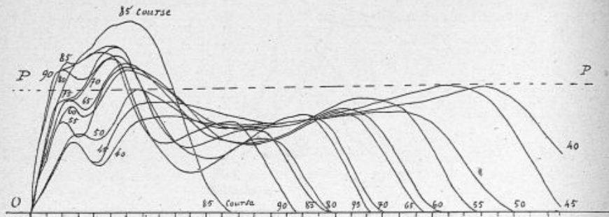
Fig. 354. — Forme de la pression normale du pied sur le sol dans des marches variant de la cadence 40 à 90.
