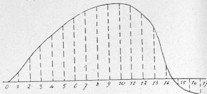
Fig. 368. — Variation de la vitesse relative du pied par rapport à la hanche dans la marche pendant le lever et projeté horizontalement. Les périodes correspondent à l'analyse cinématique de la figure 367.
