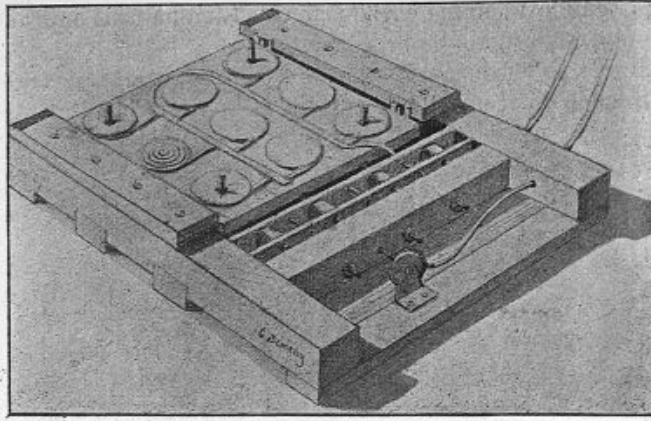
Fig. 339. — Intérieur d'un dynamographe donnant en fonctions du temps la courbe de la pression normale et tangentielle des pieds sur le sol dans les diverses allures (MAREY et DEMENY).
