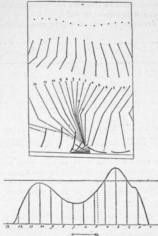
Fig. 341. — Combinaison des indications dynamographiques avec les données cinématiques de la chronophotographie.
