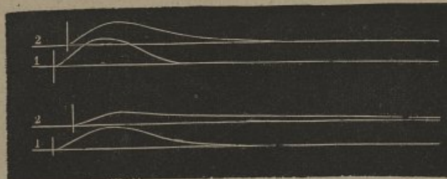
Fig. 25. Tracé du passage d'une onde musculaire.
