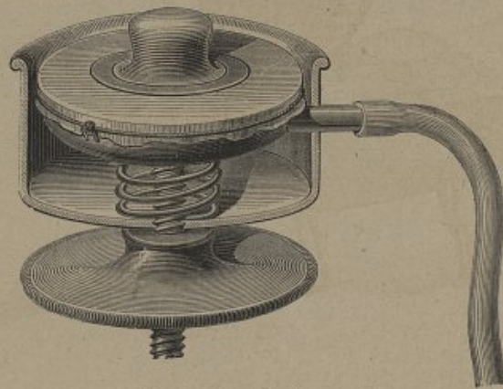
Fig. 8. Coupe de l'appareil.
