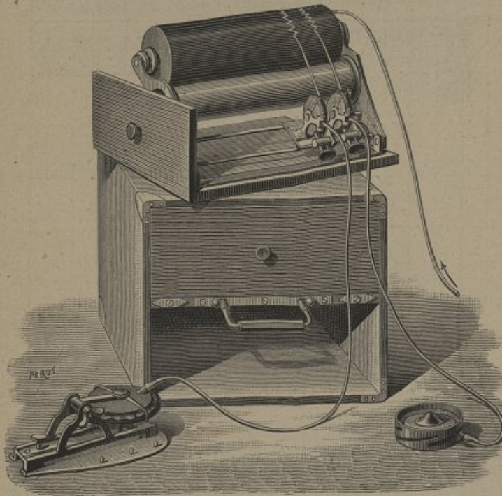
Fig. 48. Polygraphe universel.
