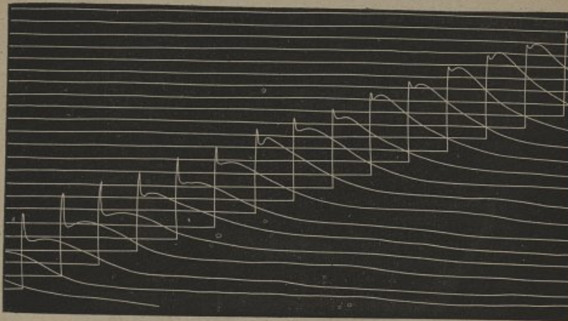
Fig. 19. Tracés imbriqués obliquement. Phases successives de l'empoisonnement d'un muscle par la vératrine.
