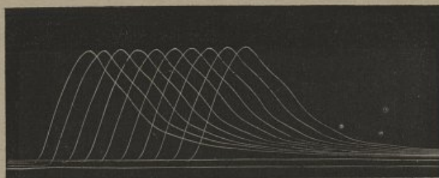
Fig. 18. Tracés du myographe simple imbriqués latéralement.
