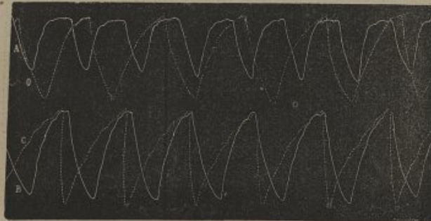
Fig. 16. Tracés des mouvements respiratoires de l'homme.
