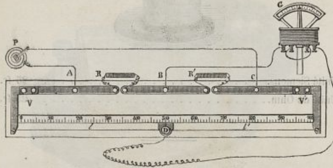
Grand appareil dit pont de Wheatstone.
