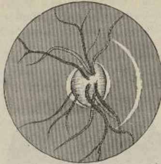
FIG. 53. — Le reflet de Weiss se présente sous la forme d'un arc argenté, à une petite distance du bord interne de la papille. Dans notre dessin cet arc est trop apparent.
