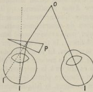
FIG. 50. — Schéma indiquant l'effet d'un prisme (base interne) dans le cas d'insuffisance des droits internes.
