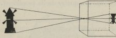
FIG. 7. — Chambre noire. L'image de l'objet se peint renversée sur la paroi opposée à l'ouverture par laquelle les rayons pénètrent.
