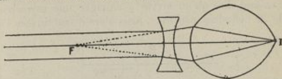
FIG. 14. — Correction d'un œil myope par un verre concave. Les rayons parallèles vont faire leur foyer sur la rétine r , comme si l'objet se trouvait en F , foyer virtuel du verre.
