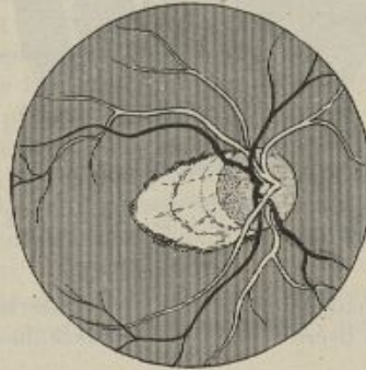
FIG. 55. — Vaste croissant ayant la forme d'un cône.
