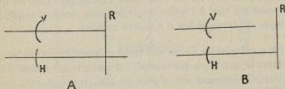
FIG. 26. — Ce schéma représente la transformation d'une astigmatie verticale hyperopique simple (A) ou astigmatie verticale myopique simple (B).
