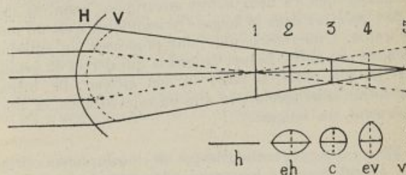
FIG. 12. — Marche des rayons lumineux dans un œil astigmat. La courbe H, à trait plein, représente le méridien horizontal d'une cornée; la courbe V, à trait pointillé, le méridien vertical. L'écran rétinien, placé successivement en 1, 2, 3, 4, 5, serait impressionné par la série des images suivantes : h, ligne horizontale; eh, ellipse; c, cercle; ev, ellipse; v, ligne verticale.
