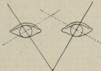
FIG. 49. — Schéma indiquant la direction la plus fréquente des astigmies. La ligne à trait plein est relative à l'astignie cornéenne, celle pointillée à l'astignie cristallinienne.
