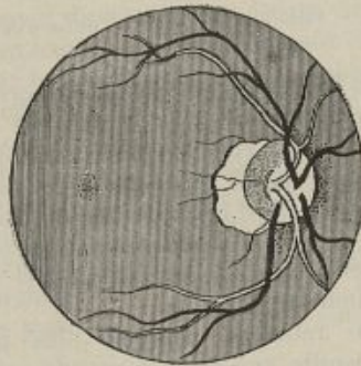
FIG. 54. — Croissant à la partie externe de la papille.
