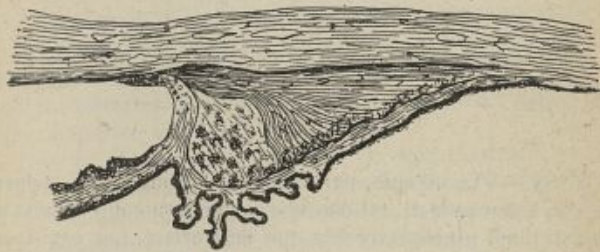
FIG. 45. — Muscle ciliaire d'un hyperope. Ces deux derniers dessins sont la reproduction de ceux donnés par Jaeger et de Wecker dans leur Atlas.
