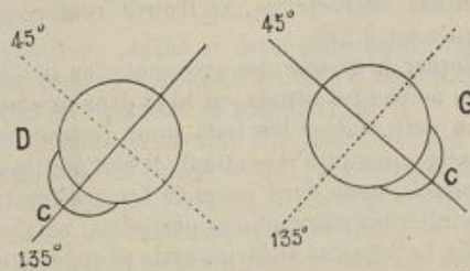
FIG. 55. — Schéma représentant la direction des croissants papillaires dans les cas d'astigmies cornéennes obliques de l'œil droit (D) sur 45 degrés et de l'œil gauche (G) sur 135 degrés. Les croissants (C, C) sont à l'extrémité externe des contractions partielles correctrices.
