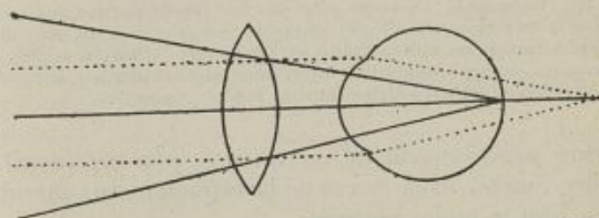
FIG. 15. — Correction de l'hyperopie à l'aide d'un verre convexe. Les rayons parallèles, au lieu d'aller se réunir au delà de la rétine, forment leur foyer sur cette membrane, exactement comme s'ils étaient pourvus d'un certain degré de convergence.
