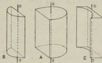
FIG. 4. — Lentilles cylindriques : A, cylindre duquel on a retranché le segment B, constituant une lentille cylindrique convexe ; C, lentille cylindrique concave ; x, y , axe du cylindre et des lentilles.
