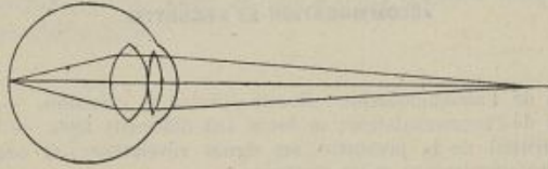
FIG. 22. — Une lentille additionnelle peut représenter l'accommodation.
