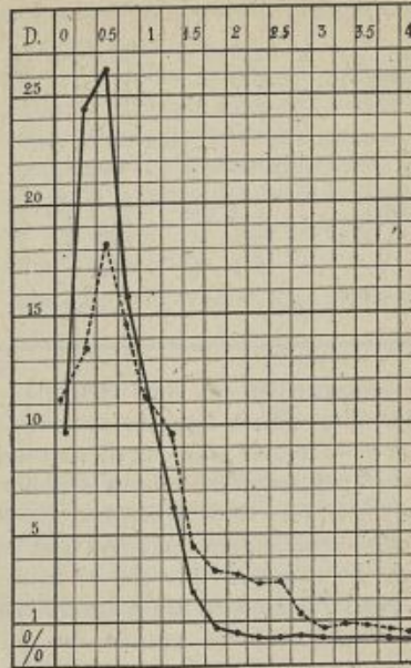
FIG. 48. — Le graphique à trait plein est relatif à l'astigmatisme cornéen des non-myopes; la ligne pointillée à celle des myopes.
