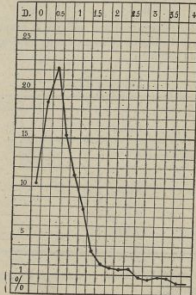
FIG. 47. — Fréquence des divers degrés de l'astigmatisme cornéen dans des yeux normaux de n'importe quelle réfraction. Les chiffres verticaux indiquent le pourcentage; les horizontaux, les degrés dioptriques.
