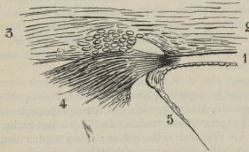
FIG. 32. — 1. La membrane de Descemet. — 2. Cornée. — 3. Sclérotique. — 4. Attache antérieure du muscle ciliaire. — 5. Iris.
