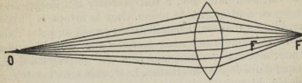
FIG. 15. — Les rayons divergents du point O, après avoir traversé la lentille biconvexe, vont faire leur image, non au foyer F, mais au delà, en F'.
