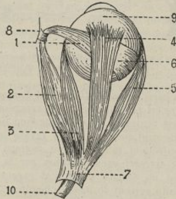
FIG. 6. — Muscles moteurs de l'œil vus par la partie supérieure de l'orbite : 1. Muscle grand oblique (portion réfléchie). — 2. Idem (portion directe). — 3. Droit interne. — 4. Droit supérieur. — 5. Droit externe. — 6. Petit oblique. — 7. Anneau d'insertion des muscles. — 8. Poulie de réflexion du grand oblique. — 9. Globe oculaire. — 10. Nerf optique.
