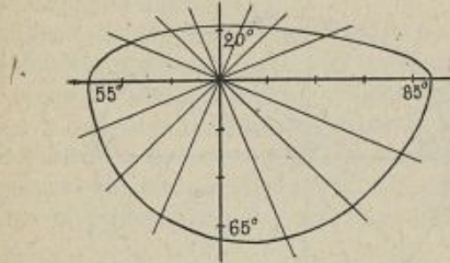
FIG. 43. — Champ visuel d'un œil droit atteint d'un décollement de la partie inférieure de la rétine : le champ visuel est rétréci en haut par suite de ce décollement.
