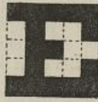
FIG. 28. — Lettre faisant partie du tableau d'épreuve; vue à 5 mètres, elle indique une acuité visuelle de \frac{1}{5} .
