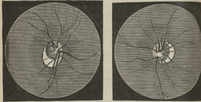
FIG. 55 et 54. — Elles représentent le fond des deux yeux d'une même personne. L'œil droit (fig. 55) présente une astigmatie horizontale et le gauche une astigmatie verticale. Dans chaque organe, le croissant se trouve donc à l'extrémité de la contraction partielle correctrice.
