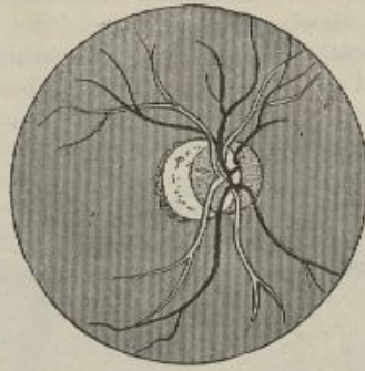
FIG. 59. — Croissant avec empiètement de la rétine sur la surface de la papille.
