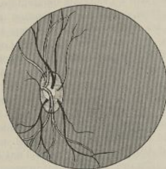
FIG. 53. — Image ophtalmoscopique représentant la direction presque verticale des vaisseaux rétiniens dans le cas d'amblyopie astigmatique monolatérale.
