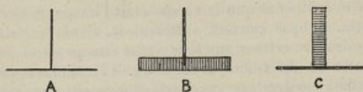
FIG. 25. — Images rétinienne dans l'astigmatisme : A, deux lignes placées à angle droit; B, leur image sur la rétine d'un astigmatisme selon la verticale; C, leur image lorsque l'astigmatisme est horizontale.
