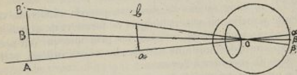
FIG. 27. — Angle visuel d'objets de grandeur et d'éloignement différents.
