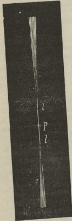
FIG. 25. — Point d'accommodation ( p ) et ligne d'accommodation ( l , l ).
