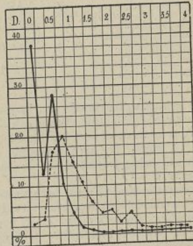
FIG. 51. — Graphique de l'astigmatisme subjectif des non myopes (ligne pleine), des myopes (ligne pointillée).
