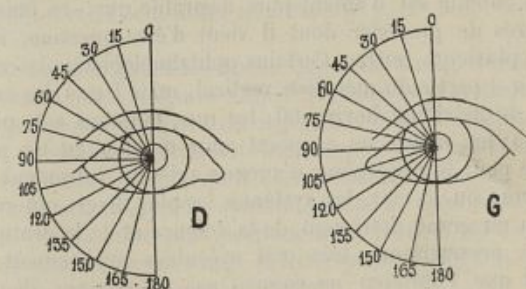
Fig. 19. — Graduations des méridiens de l'œil ; elle est la même pour les deux yeux.
