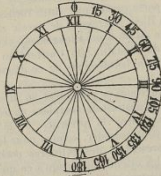
Fig. 17. — Cadran horaire pour la détermination de l'astigmatisme. Les lignes noires, espacées de 15 degrés, correspondent aux heures et demi-heures. La graduation commence au méridien vertical (midi) et marche dans le sens des aiguilles. Réduction au 1/10.
