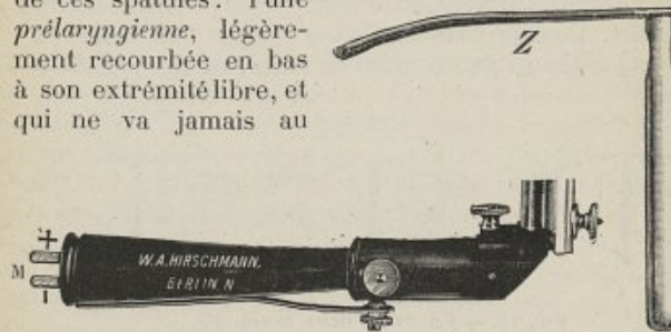
Fig. 27 et 28. — Laryngoscope de Kirstein.
