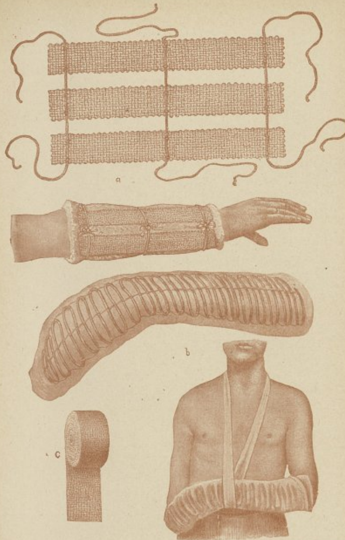
a , Toile métallique d'Esmarch; b , Attelles de fil de fer en spirale de Heusner; c , Bandes métalliques roulées de Port.
