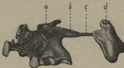
Fig. 75. — Obturateur palatin de Schlitsky, légèrement modifié. a, plaque dentaire ; b, partie métallique ; c, ressort à boudin ; d, plaque de caoutchouc mou.
