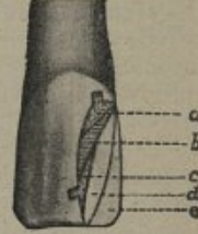
Fig. 135. — Marche d'une aurification à l'or cohésif dans une cavité approximale de grandes dimensions d'une incisive: a , or cristallisé et petits cylindres; b , grands cylindres; c , or cristallisé et petits cylindres; d , grands cylindres (peu flambés); e , feuille d'or n° 40 (fortement flambée).
