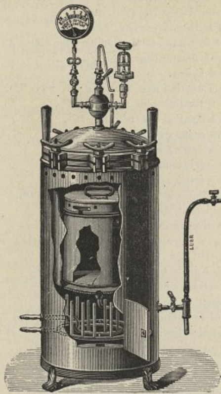
Fig. 7. — Autoclave de Chamberland.
