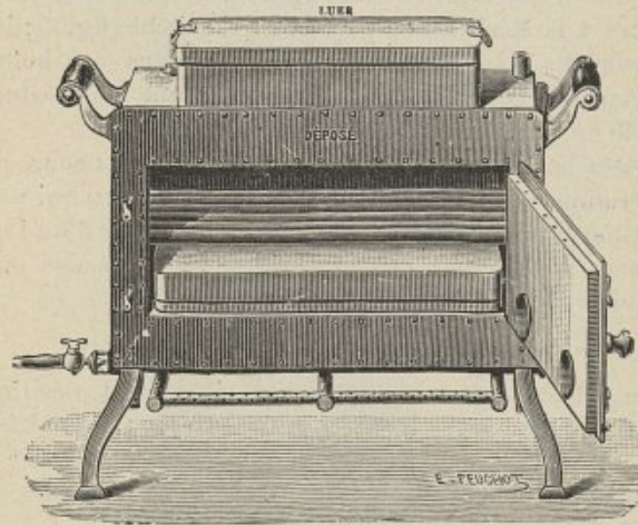
Fig. 6. — Stérilisateur à air sec de Poupinel.
