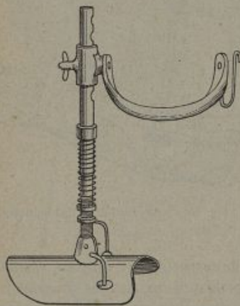
Fig. 56. — Appareil de Leclercq.
