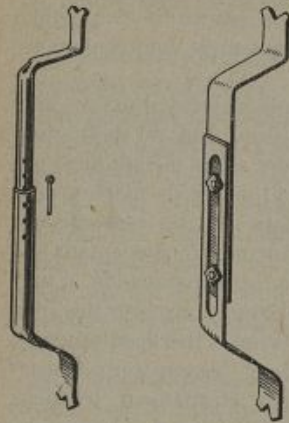
Fig. 56. — Anses de feuillard à coulisses et à écrous.
