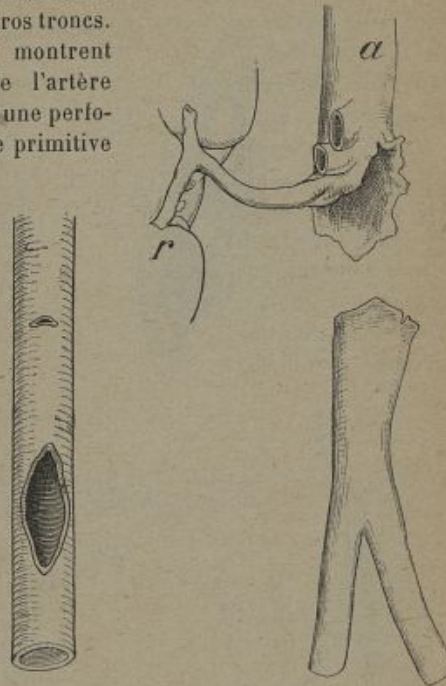
FIG. 2. (schématique). Deux plaies latérales d'une artère.
