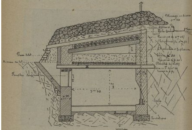
Fig. 55. — Mode de protection d'un abri pour l'exercice de la chirurgie d'urgence à l'avant, près du front. TISSERAND [47].
