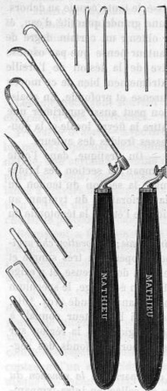
Fig. 101. — Variétés de ténotomes à manche coudé.
