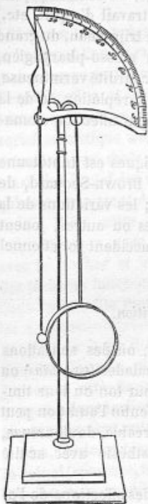
Fig. 145. — Acoumètre d'Itard, une boule métallique est écartée d'une distance indiquée au moyen du cadran, et vient frapper un anneau métallique ; le son est ainsi produit avec une intensité calculable.
