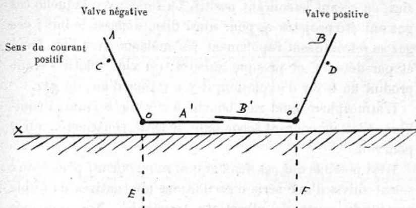
Fig. 2. — Deux soupapes à air montées pour chute en recouvrement. Schéma en profil.
