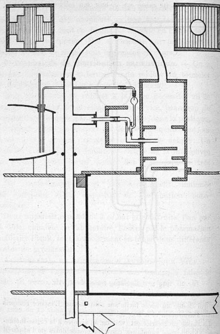
Fig. 5. — Appareil de distribution automatique de M. Vila.
