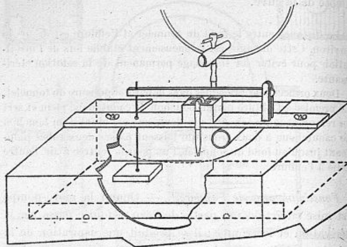
Fig. 6. — Appareil de distribution automatique du pharmacien-auxiliaire Piault.
