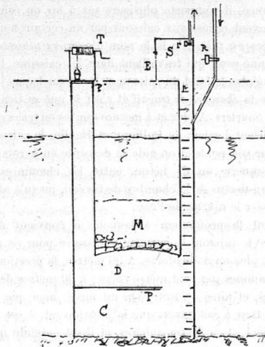
Fig. 1. — Schéma d'un caisson.
