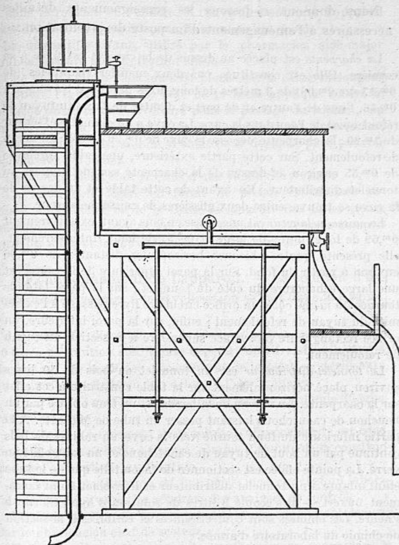
Fig. 2. — Poste de javellisation. — Modèle du Laboratoire de bactériologie et de chimie de la .. e armée (d'après le travail de M. Orticoni).
