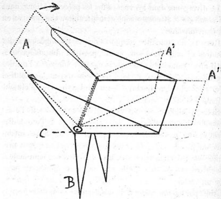
Fig. 1. — Soupape à air.
