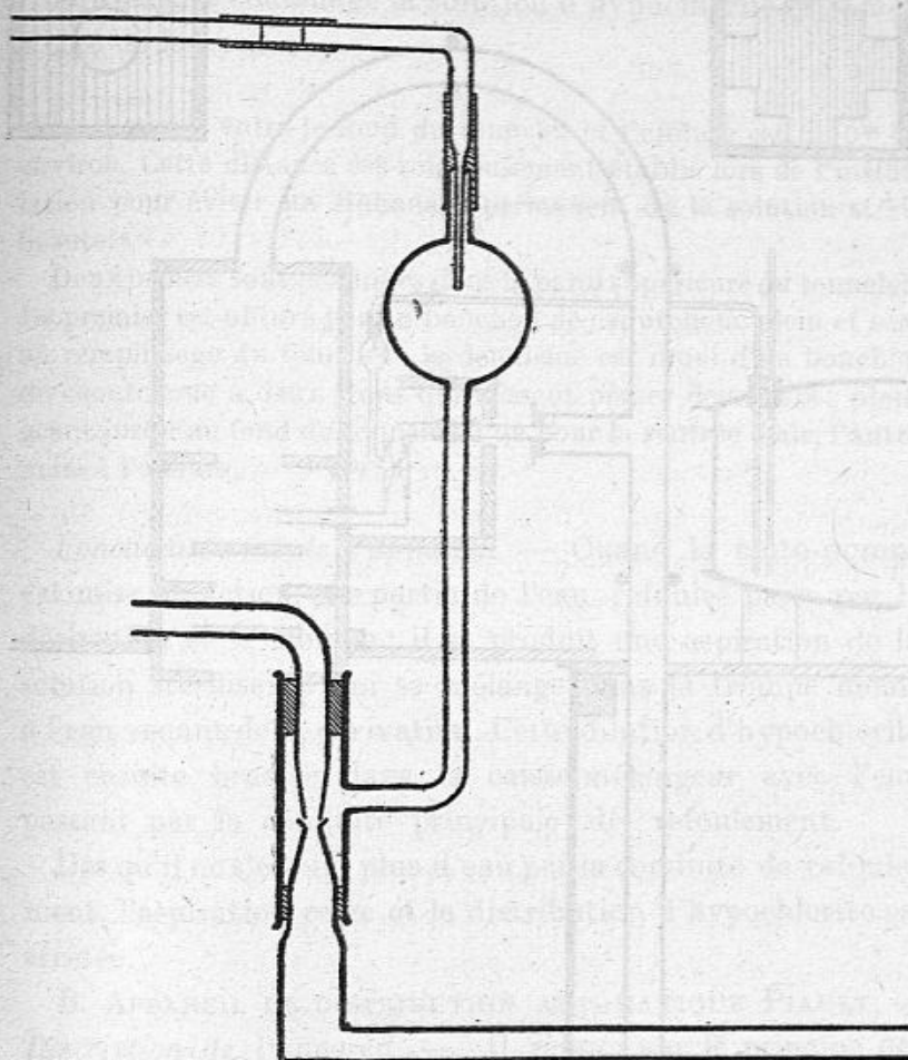
Fig. 4. — Aspirateur-trompe de M. Vila.
