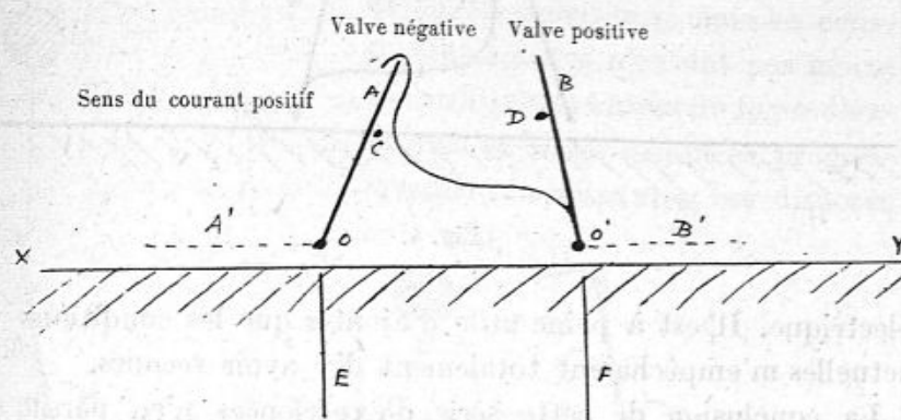
Fig. 3. — Deux soupapes à air montées en couple dépendant.
