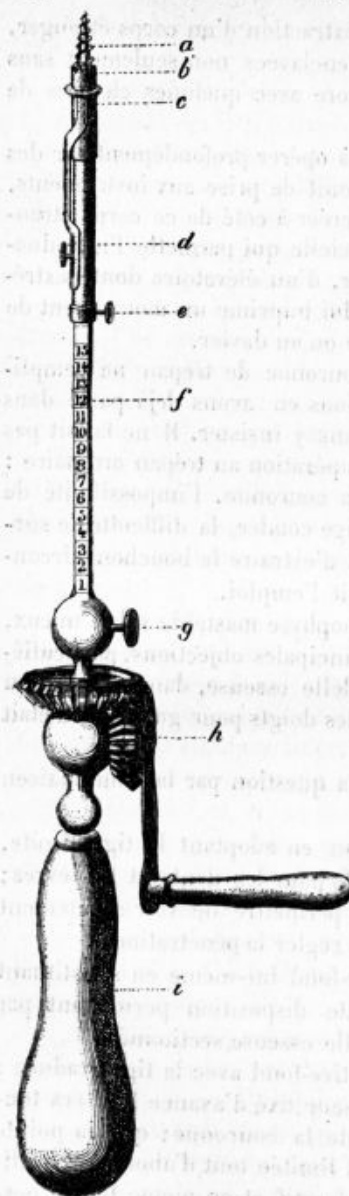
Trépan-tire-fond (1/2 grandeur)
