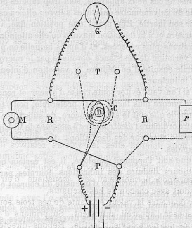
Fig. 1. — Pont différentiel disposé pour la mesure des excitants.
