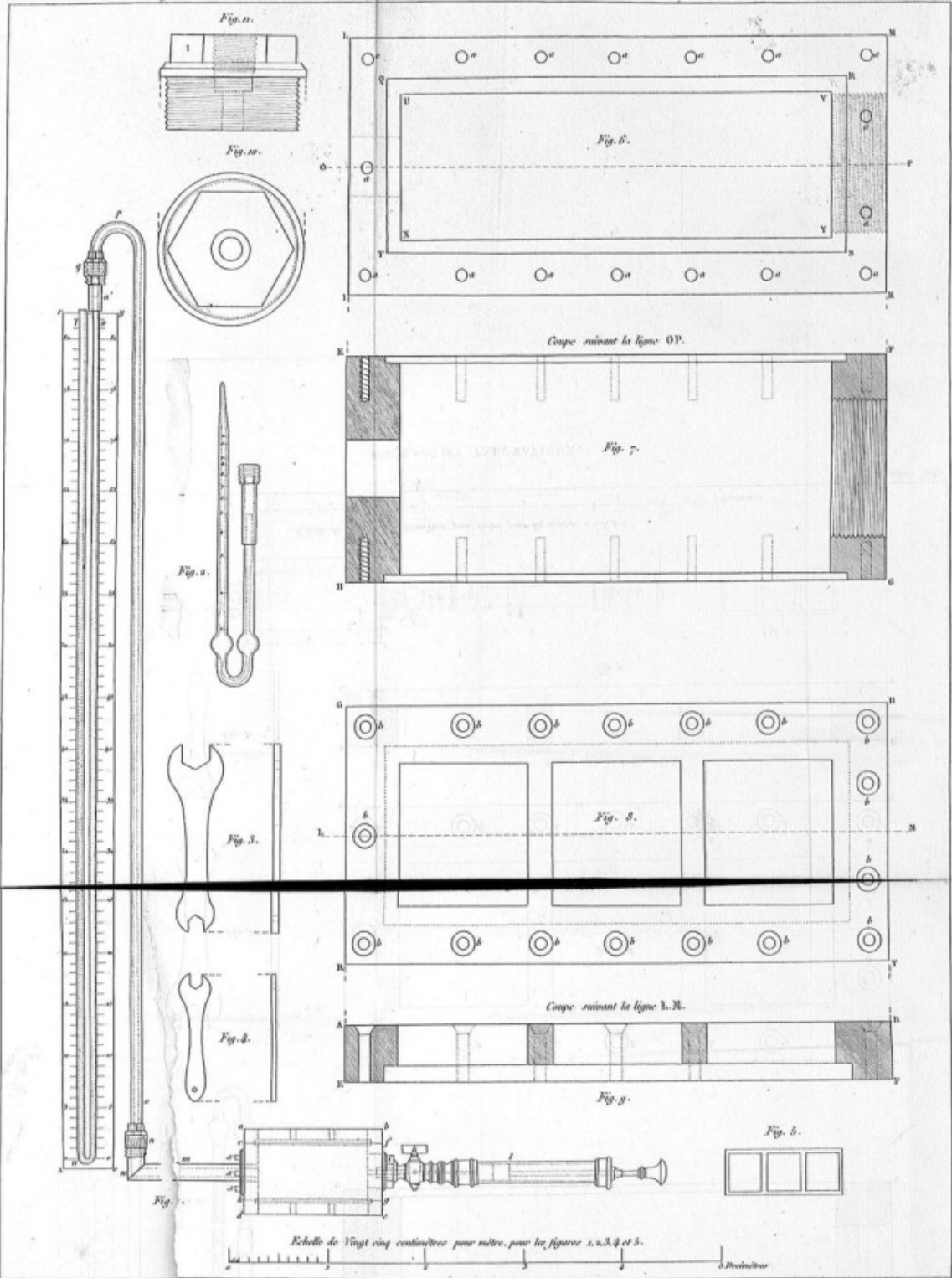
PORTE-OBJET PNEUMATIQUE.
