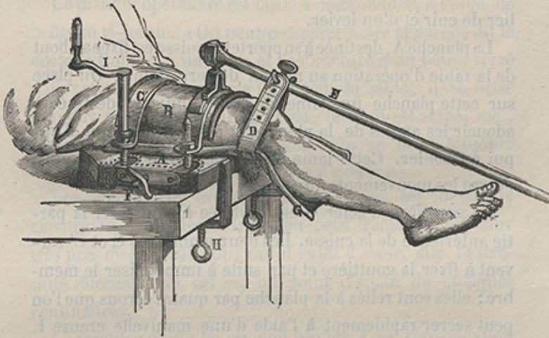
Fig. 8. — Ostéoclaste du docteur Robin.
