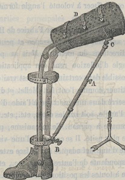
Fig. 2. — Appareil de Mathieu.
