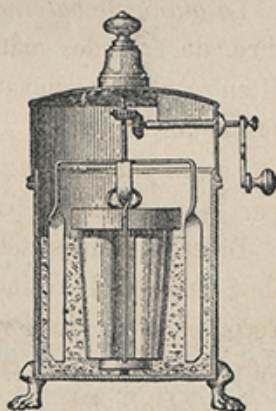
FIG. 1. Glacière domestique 1.
