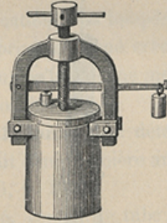
FIG. 10. Marmite de Papin.
