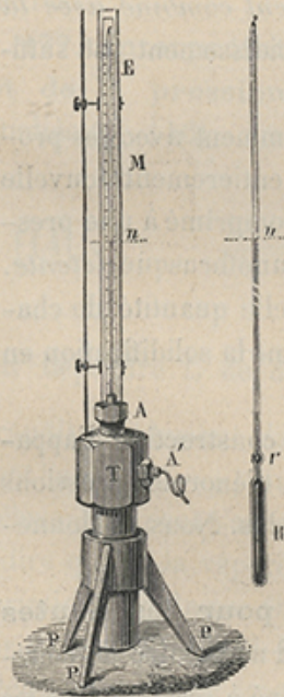
FIG. 23. Manomètre fondé sur l'élasticité du verre.
