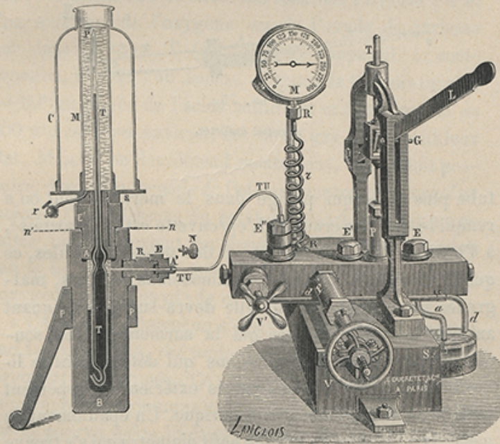
FIG. 24. Appareil Cailletet.
