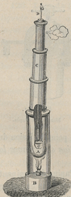
FIG 11. Hypsomètre.
