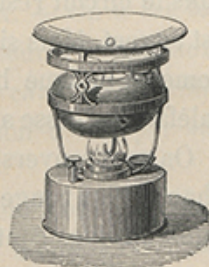
FIG. 9. Caléfaction.
