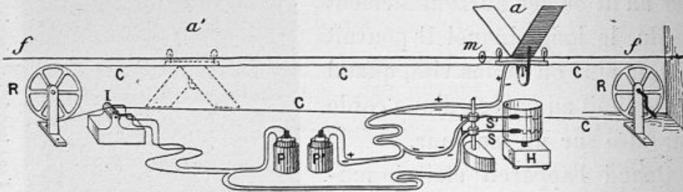
Fig. 134. — Disposition de l'expérience destinée à mesurer les durées du coup d'aile pendant une translation rectiligne plus ou moins rapide.
