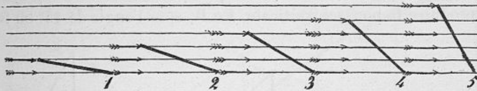
Fig. 122. — Figure théorique montrant que la résistance de l'air à un plan incliné est proportionnelle au sinus de l'angle que ce plan forme avec la direction du mouvement.
