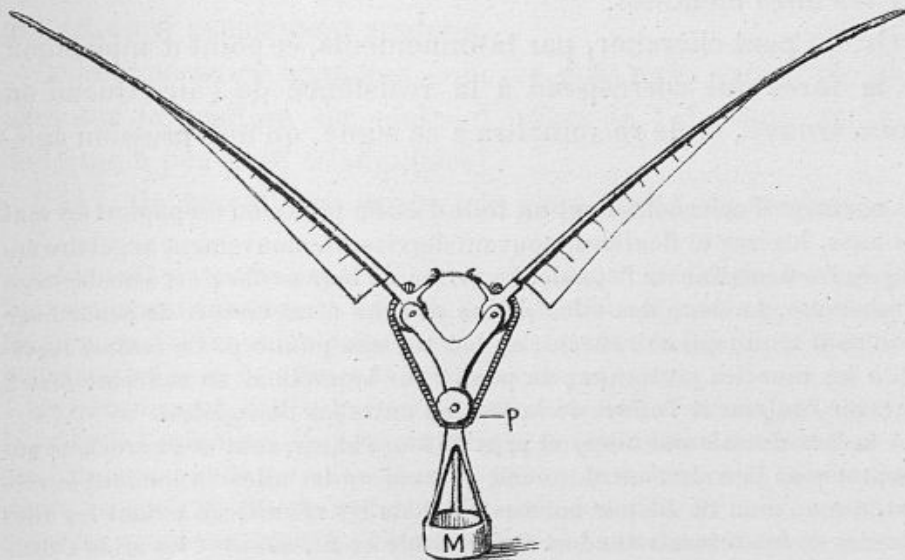
Fig. 126. — Appareil imitant le coup d'aile de l'oiseau.
