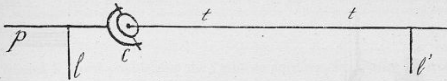
Fig. 58. — Représentation schématique du levier pantographique transmettant les changements de position de l'aile et les changements d'inclinaison de sa surface.
