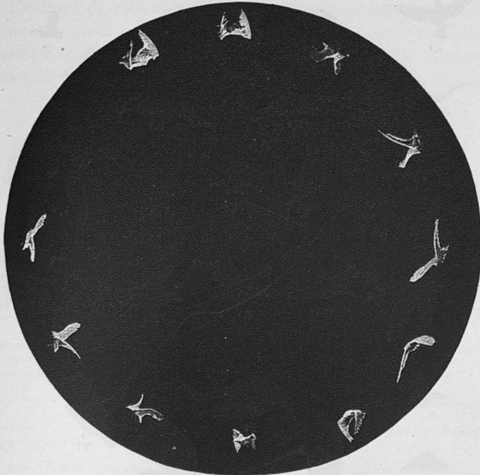
Fig. 70. — Épreuve positive du fusil photographique montrant une Mouette qui vole dans la direction de l'observateur. L'oiseau se détache sur un fond obscur, ce qui fait que ses images présentent un certain modelé au lieu d'une simple silhouette. Une imperfection dans la visée a fait que la douzième image ne s'est pas produite.
