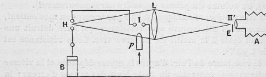
Fig. 117. — Disposition de l'appareil de Mach pour photographier les projectiles en mouvement.
