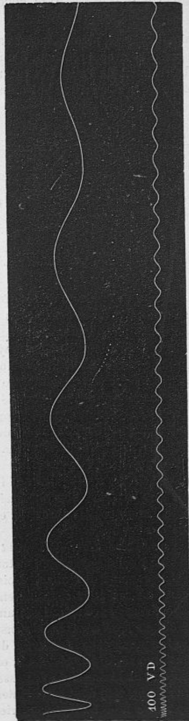
Fig. 133. — Décroissement de l'amplitude du coup d'aile d'un oiseau mécanique, sous l'influence d'une translation circulaire de l'appareil.
