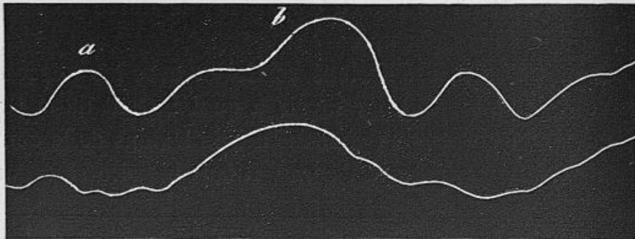
Fig. 65. — Tracés simultanés des contractions des muscles pectoraux de la Buse et des oscillations verticales de l'oiseau.
