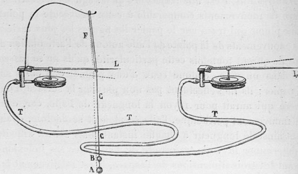
Fig. 49. — Tambours à leviers conjugués.
