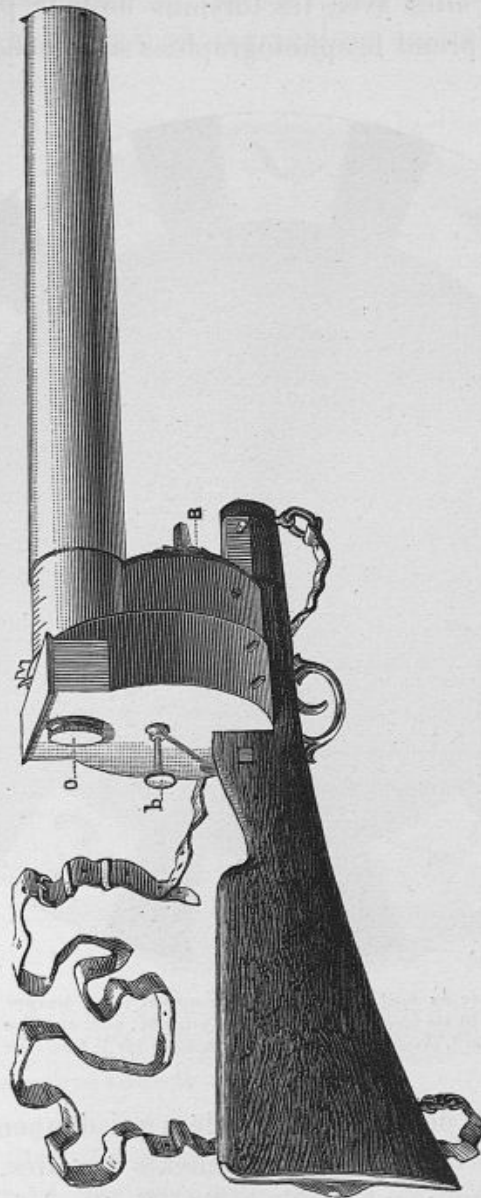
Fig. 68. — Le fusil photographique.
