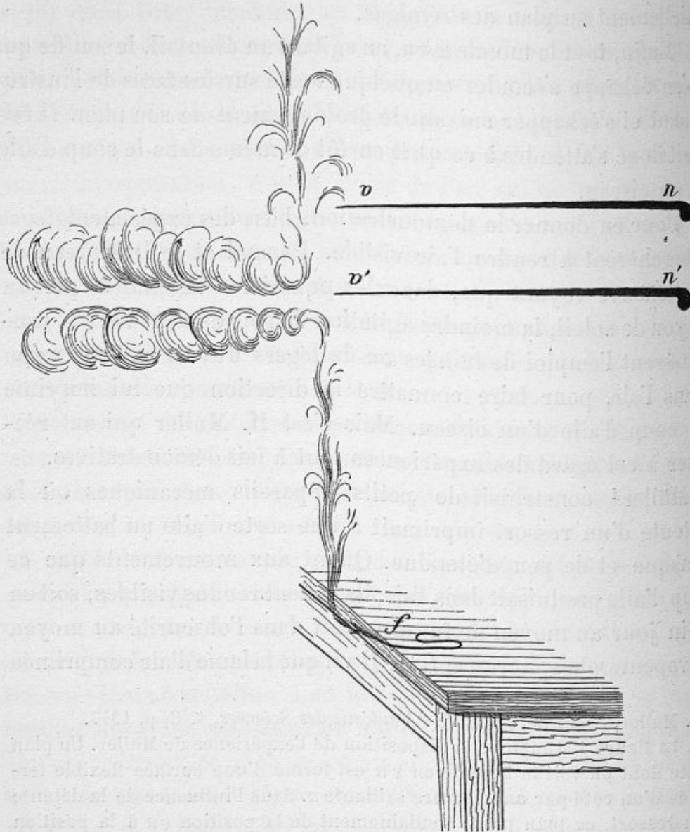
Fig. 138. — Expérience de Müller montrant les mouvements de l'air sous l'influence du coup d'aile. La surface aliforme vn est brusquement portée en v'n' . La colonne de fumée qui montait verticalement du fil f brûlant dans l'air calme est coupée à angle droit par une lame d'air qui s'échappe du côté du voile mince de l'aile; au-dessus et au-dessous de cette nappe d'air, la fumée roule en tourbillons de sens contraire, comme le montre la direction des flèches.
