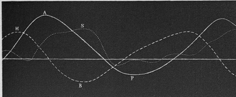
Fig. 60. — Trois courbes recueillies simultanément sur une Buse et correspondant, l'une HB aux mouvements d'élévation et d'abaissement de l'aile, l'autre AP à ses mouvements d'avant en arrière, la troisième S à sa torsion suivant son axe.
