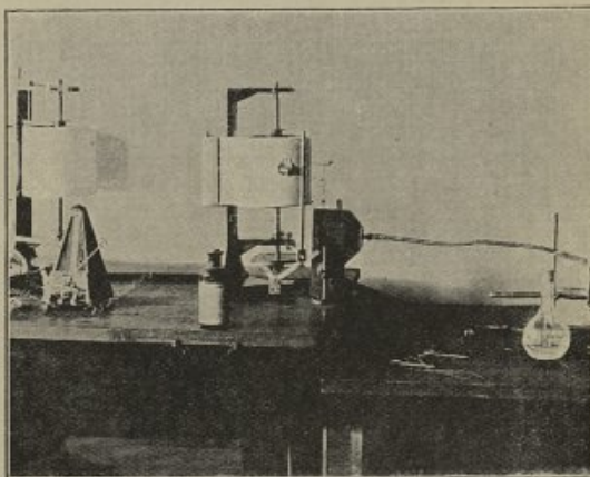
Kymographe Ludwig modifié destiné à enregistrer le résultat de l'influence des drogues sur la pression du sang, sur le cœur et la respiration.
