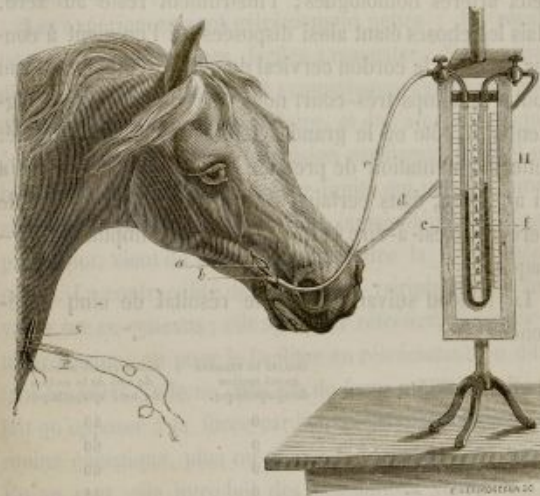
FIG. 6. — Nanomètre différentiel.
