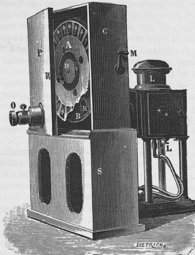
FIG. 204.—Demeny's photophone.
