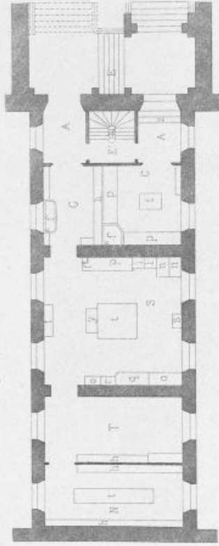
Fig. 1. PLAN DU REZ-DE-CHAUSSÉE
