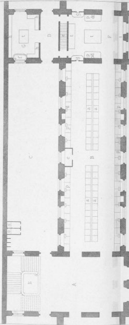
Fig. 2. PLAN D'UN LABORATOIRE DE 1 re ANNÉE (REZ-DE-CHAUSSEE)
