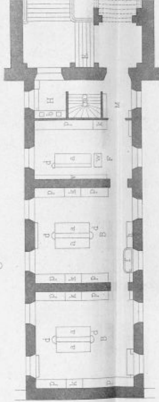
Fig. 2. PLAN DU 1 er ÉTAGE
