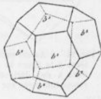
Fig. 18. — Cubo-octaèdre.
