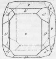
Fig. 20. — Cubo-dodécaèdre.
