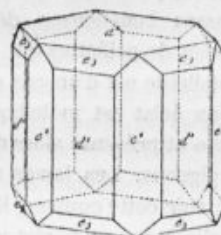
Fig. 16. — Framont.
