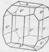
Fig. 19. — Dodécaèdre pentagonal.
