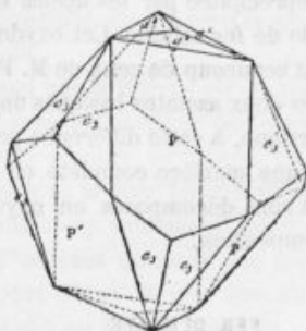
Fig. 12. — Ile d'Elbe.
