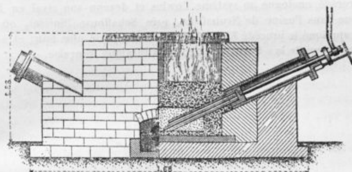
Élévation et coupe longitudinale.
