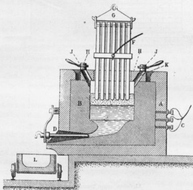
A. Boîte en fer. — B. Bloc de charbon. — C. Électrodes. — D. Trou de coulée. — E. Tampon. — F. Baguettes de charbon formant pôles. — G. Chape. — H. Couvercle du creuset. — J. Trous de chargement. — K. Couvercles de J. — L. Poche.
