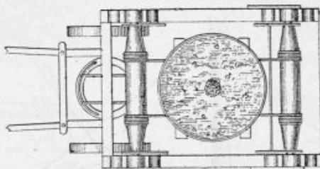
Fig. 142. — Plan du petit chariot.
