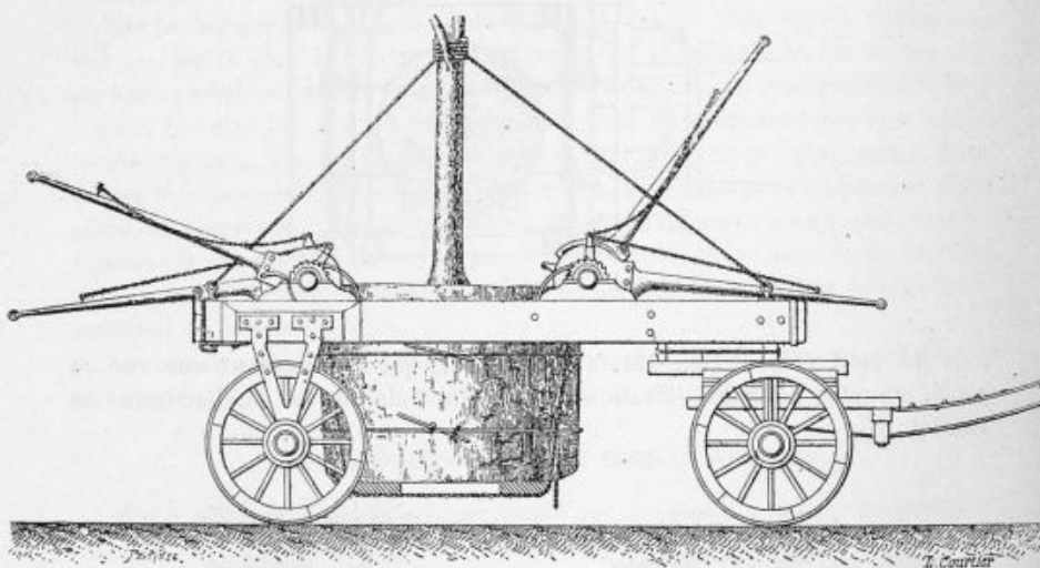
Fig. 145. — Vue de profil du chariot à deux chevaux.
