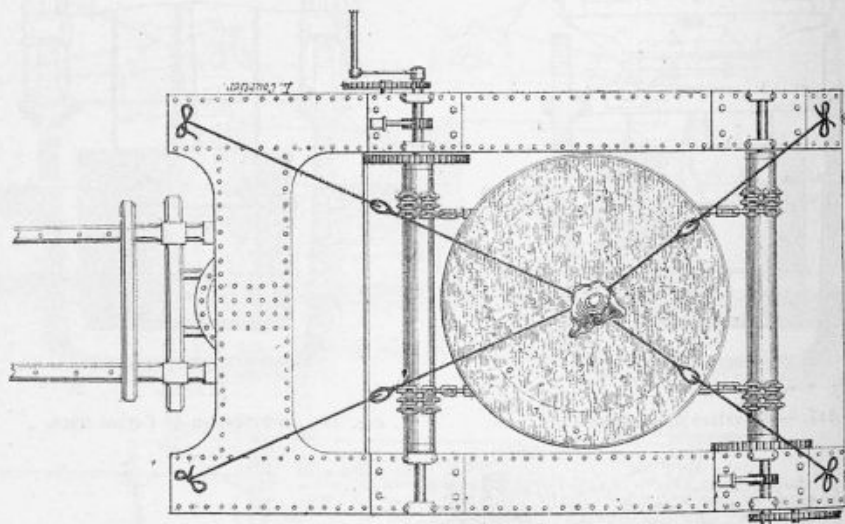
Fig. 130. — Plan du grand chariot.
