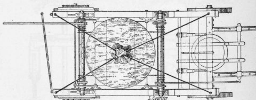
Fig. 146. — Plan du chariot à deux chevaux.
