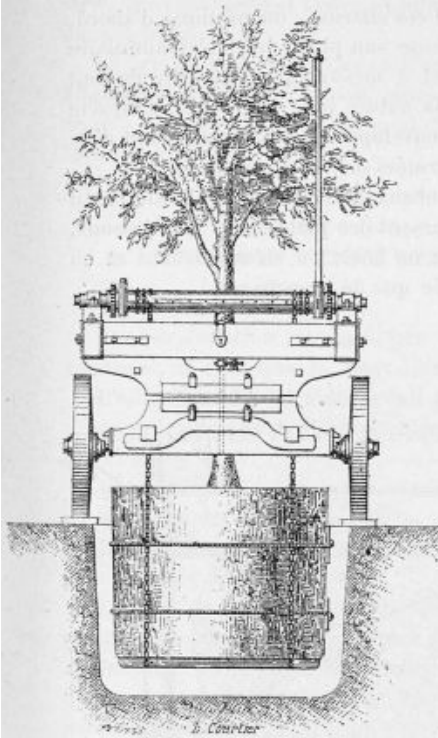
Fig. 147. — Elévation de l'arrière-train.
