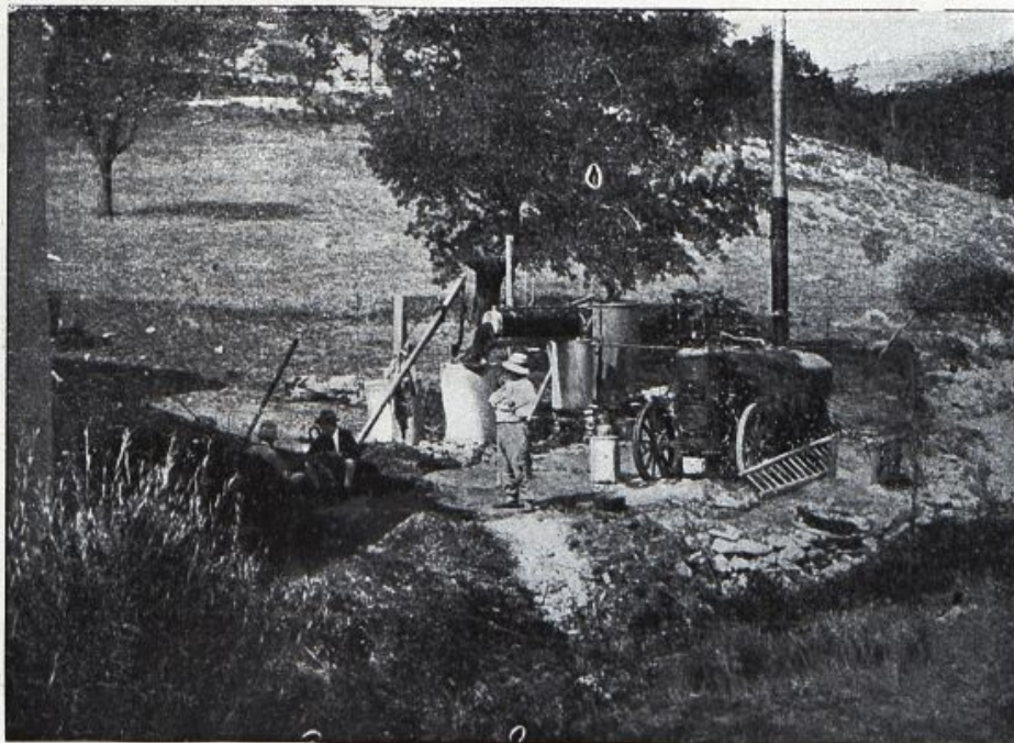
DISTILLERIE A VAPEUR SYSTEME J. M. V. A FERRASSIERES
