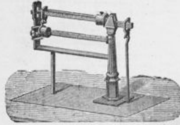
Fig. 26. Appareil démonstratif à double romaine.
