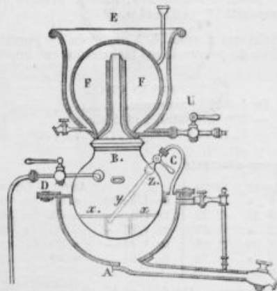
Fig. 1. Coupe de l'appareil.
