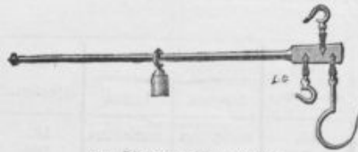
Fig. 27. Romaine oscillante.
