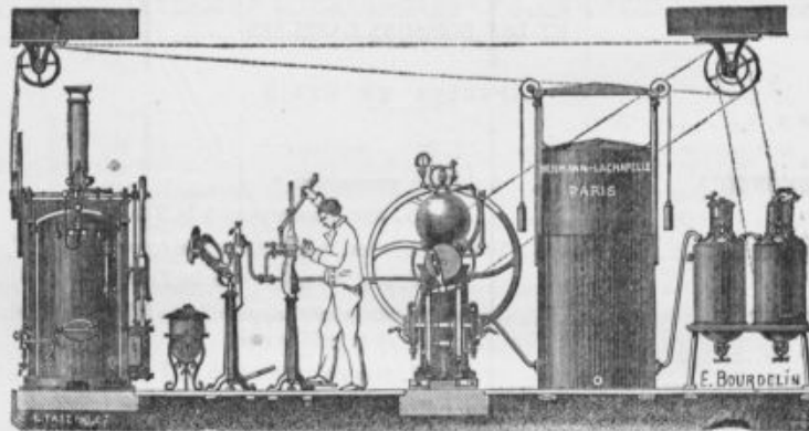
Machine à vapeur. Bassine pour sirops. Tirages. Saturateur à deux corps de pompe. Gazomètre. Épurateur et Producteur.
