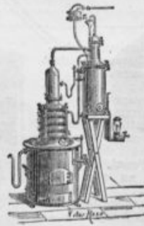
Petit Appareil Egrot à distillation continue, prêt à fonctionner. Établi de 5 grandeurs différentes pouvant produire 90° de premier jet
