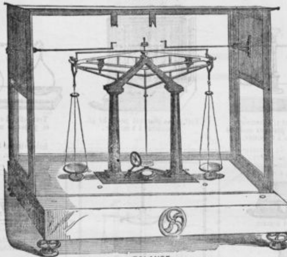
BALANCES D'ANALYSE Modèle plus simple, portée de 250 gr., et 200 gr. sensible au 1/2 mill. Prix : 210, 245, 270 et 300 fr. Envoi de dessin sur demande.
