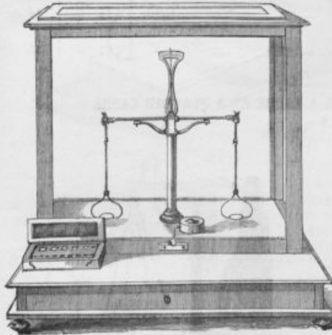
Fig. 19. Balance pour les essais d'or et d'argent.
